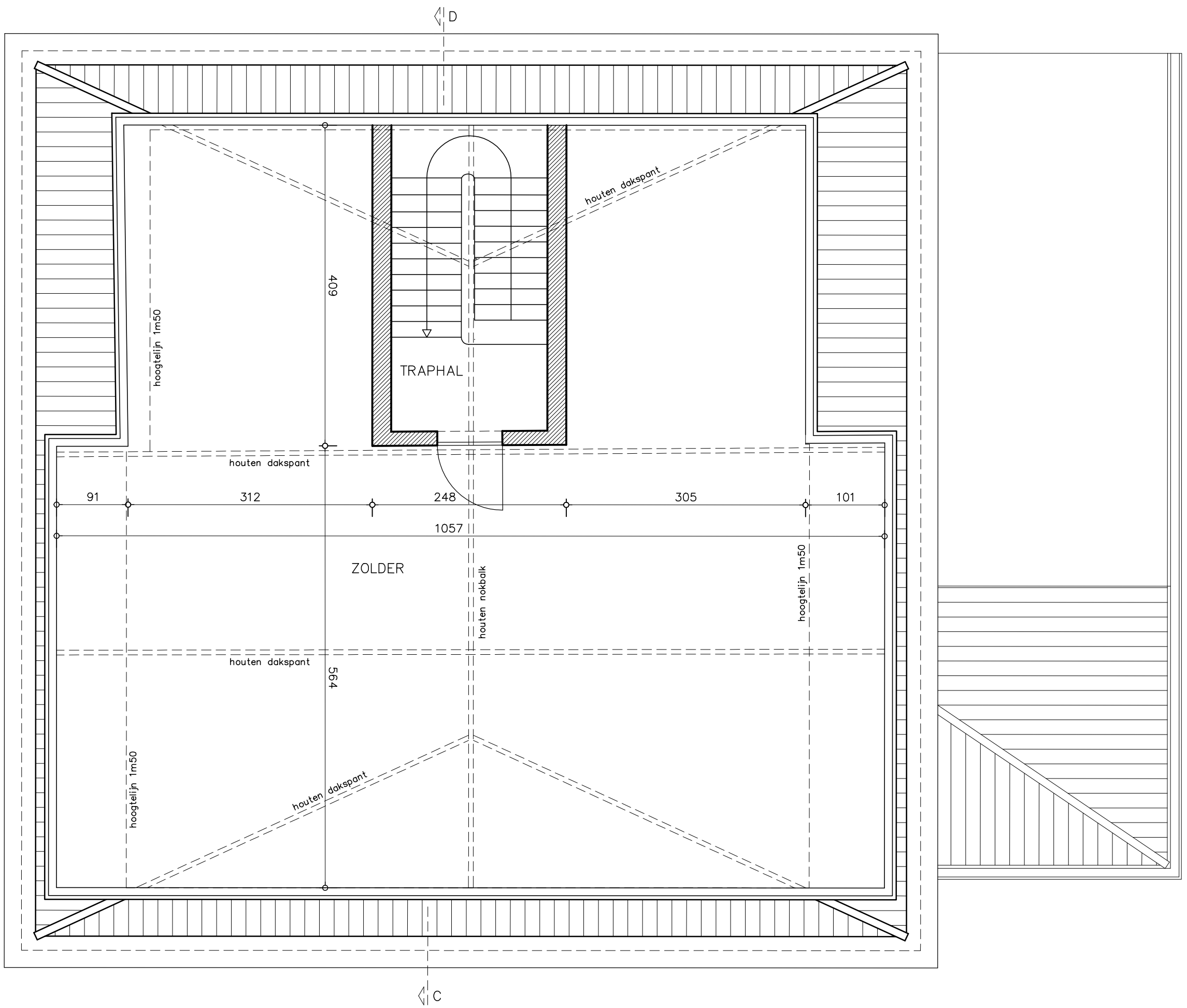
GRONDPLAN DAKVERDIEPING vergunde toestand
