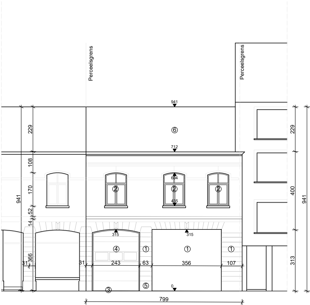
VOORGEVEL SINT ANNASTRAAT bestaande toestand
