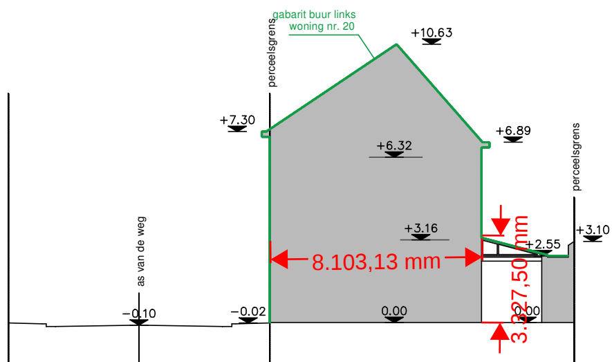
TERREINPROFIEL T2 BESTAANDE TOESTAND schaal 1/200
