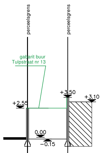
TERREINPROFIEL T3 NIEUWE TOESTAND schaal 1/200
