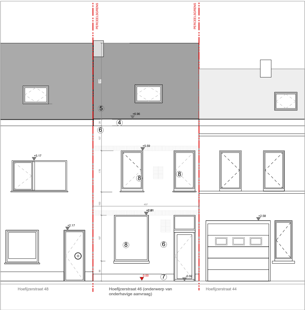
VOORGEVEL GEEN WIJZIGINGEN AAN VOORGEVEL
