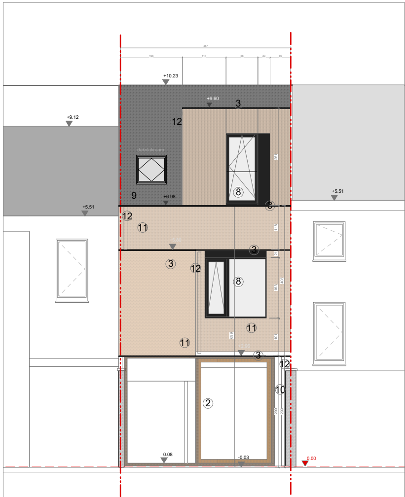
ACHTERGEVEL VERNIEUWING DAKBEDEKKING + DAKKAPEL + GEVELISOLATIESYSTEEM 15cm
