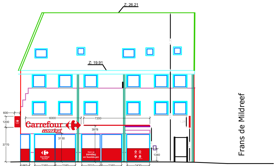
Voorgevel 2 (noord-oostgevel)
