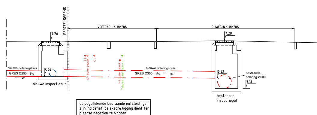
Detailtekening aansluiting riolering Glasgowstraat
