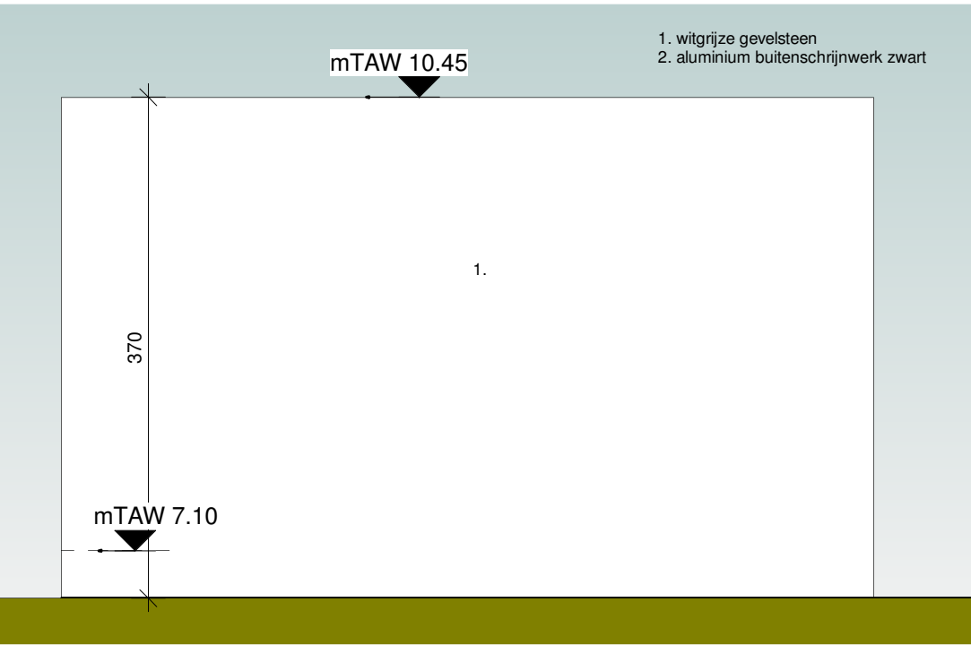
OMV Tuinberging zijgevel links 1 : 50
