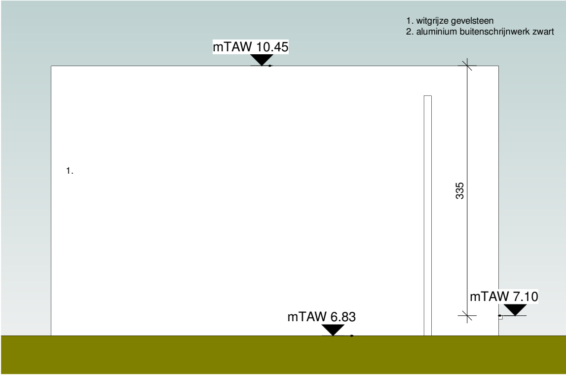
OMV Tuinberging voorgevel 1 : 50
