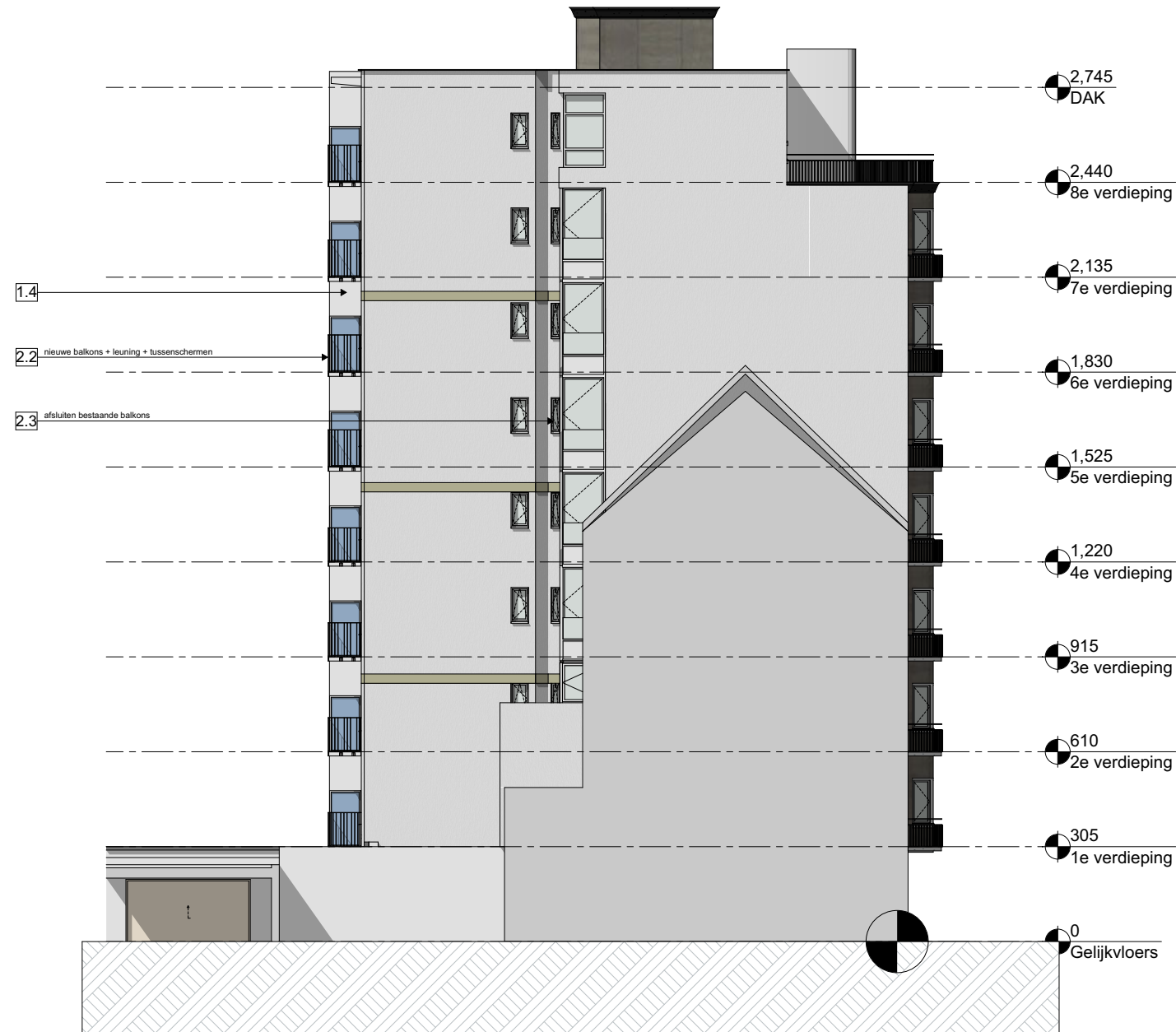
Maateenheid: Centimeter Zijgevel Links NT Schaal : 1:200 0 1 2 3 5 m
