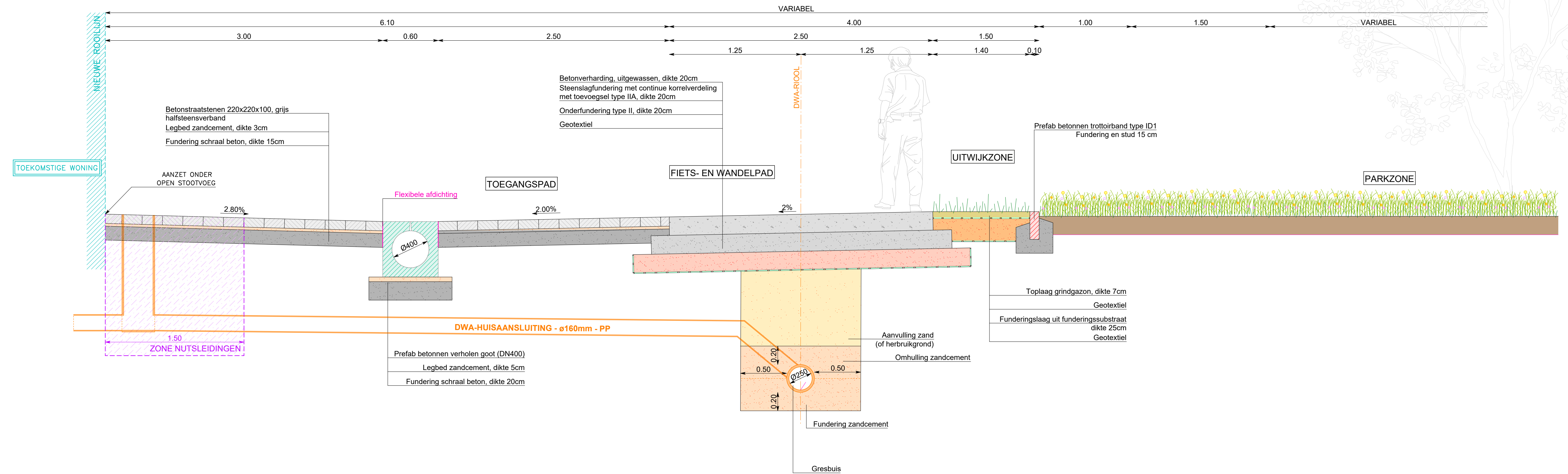
TYPEDWARSPROFIEL 01
