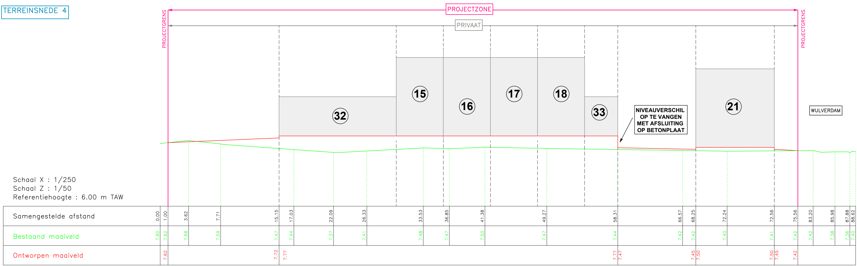
TERREINSNEDE 4
