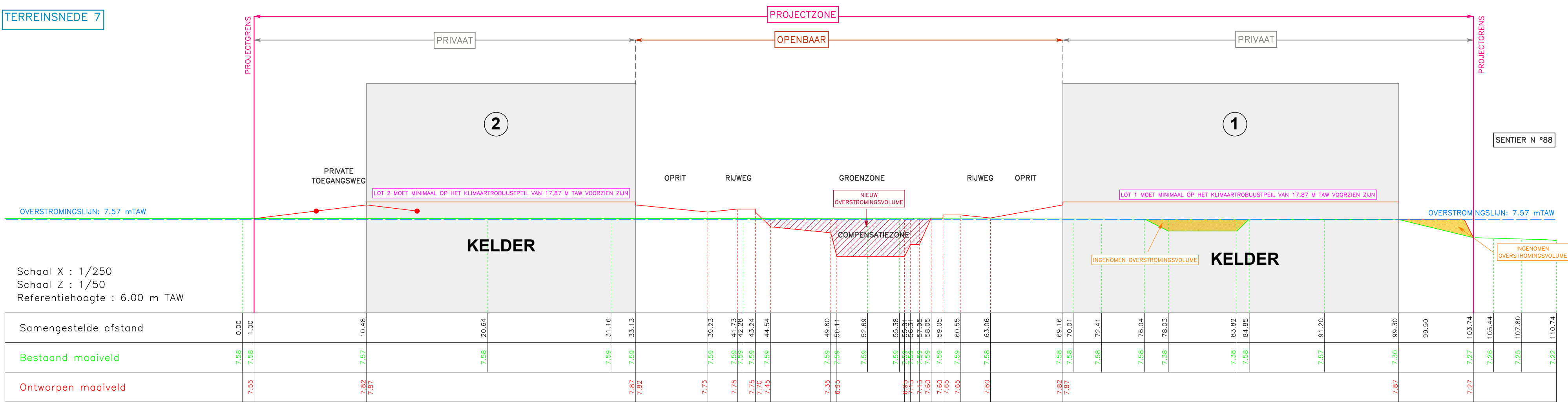
TERREINSNEDE 7
