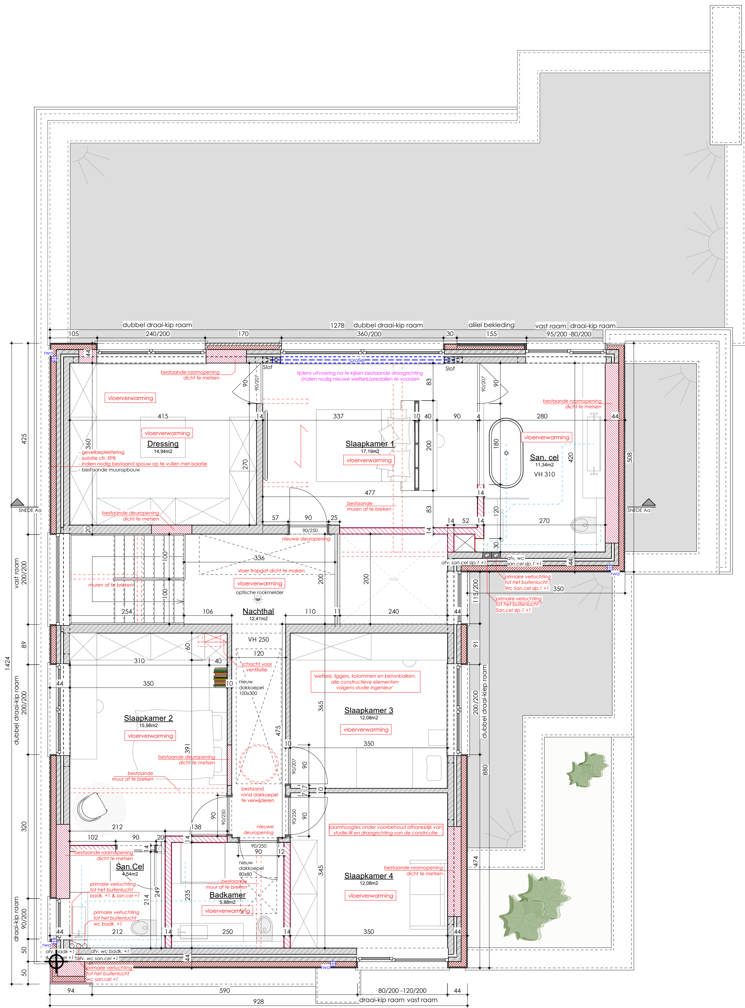
Verdiepingsplan - Bestaande toestand = Nieuwe toestand (te regulariseren) Schaal: 1:50
