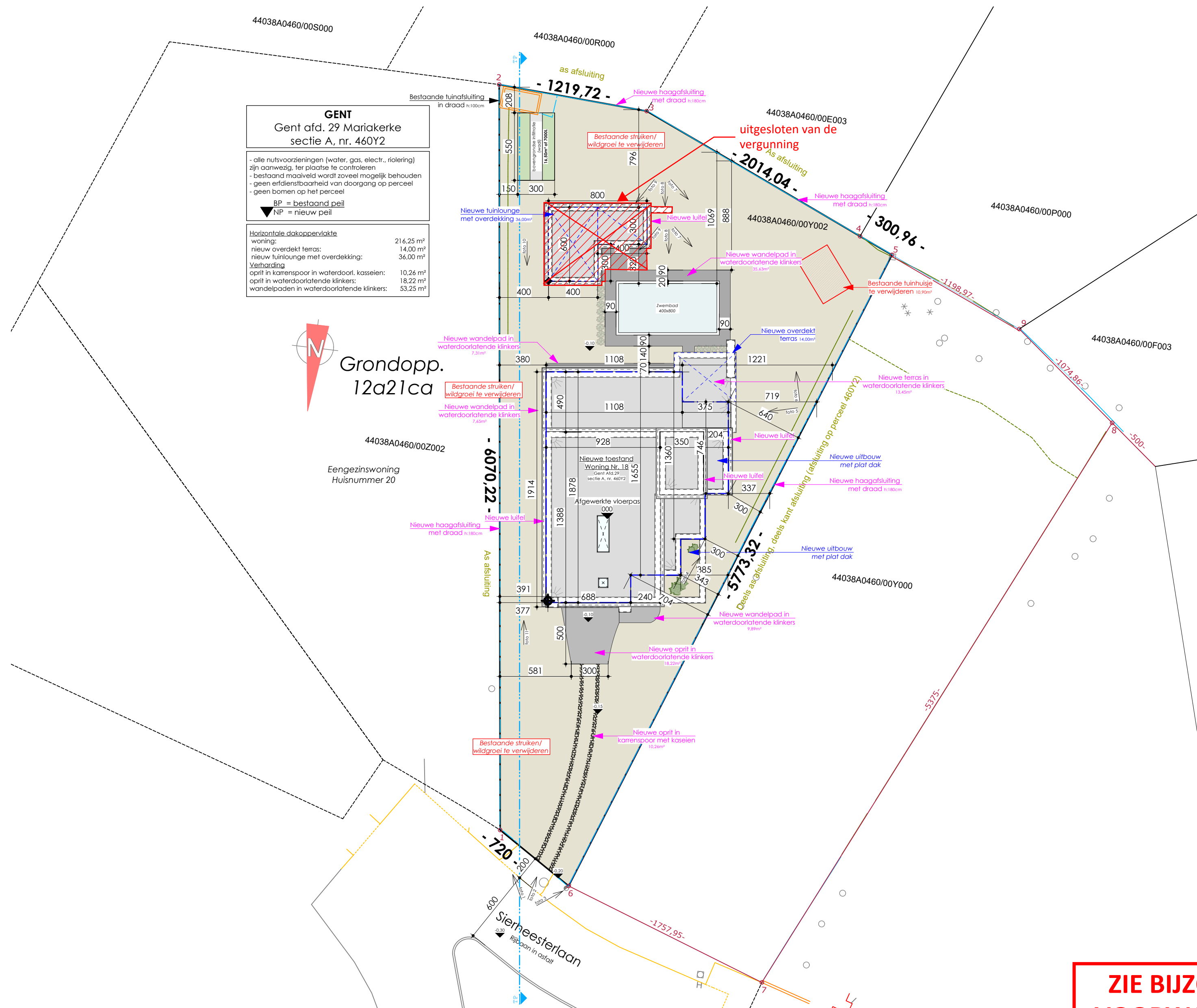
Inplantingsplan - Bestaande toestand = Nieuwe toestand (te regulariseren) Schaal: 1:250
