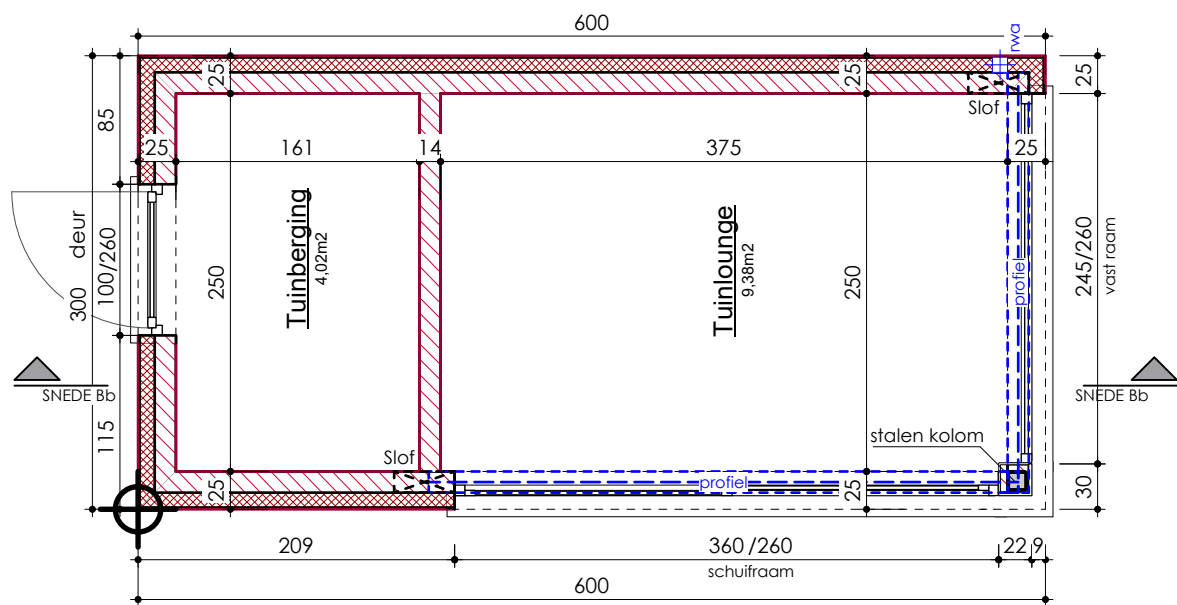
Tuinlounge met tuinberging - Vergunde toestand Schaal: 1:50
