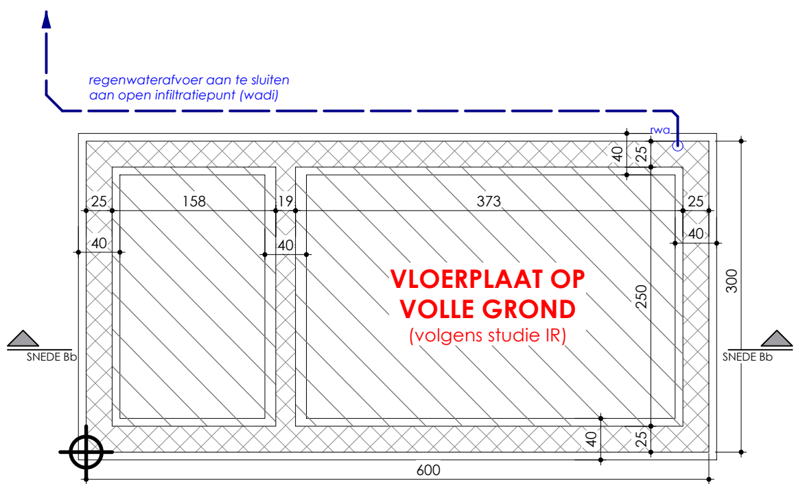
Fundering Tuinlounge met tuinberging - Vergunde toestand Schaal: 1:50
