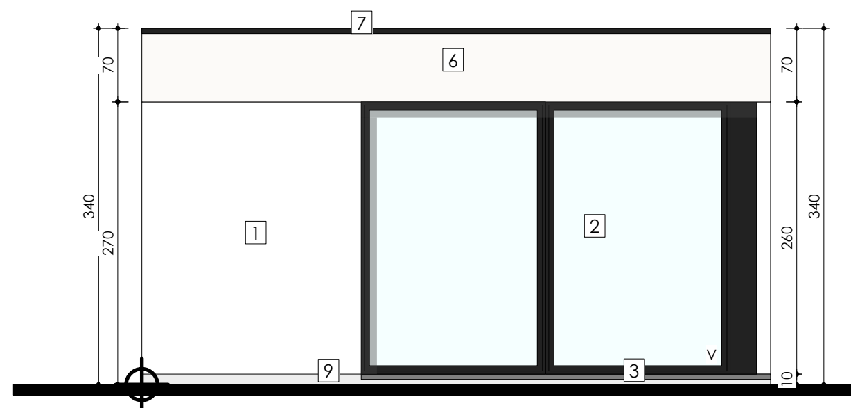
Voorgevel Tuinlounge met tuinberging - Vergunde toestand Schaal: 1:50
