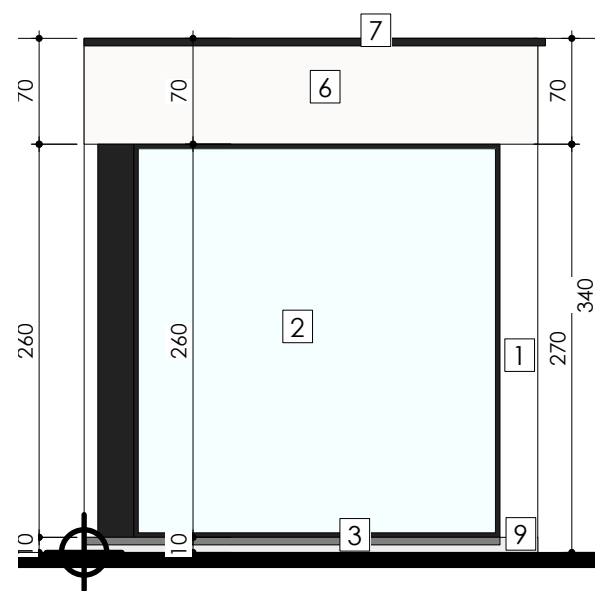
Rechter zijgevel tuinlounge met tuinberging - Vergunde toestand Schaal: 1:50
