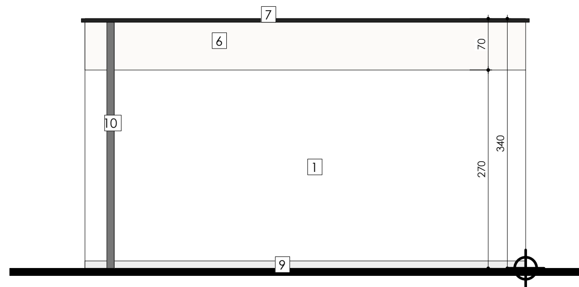
Achtergevel tuinlounge met tuinberging - Vergunde toestand Schaal: 1:50
