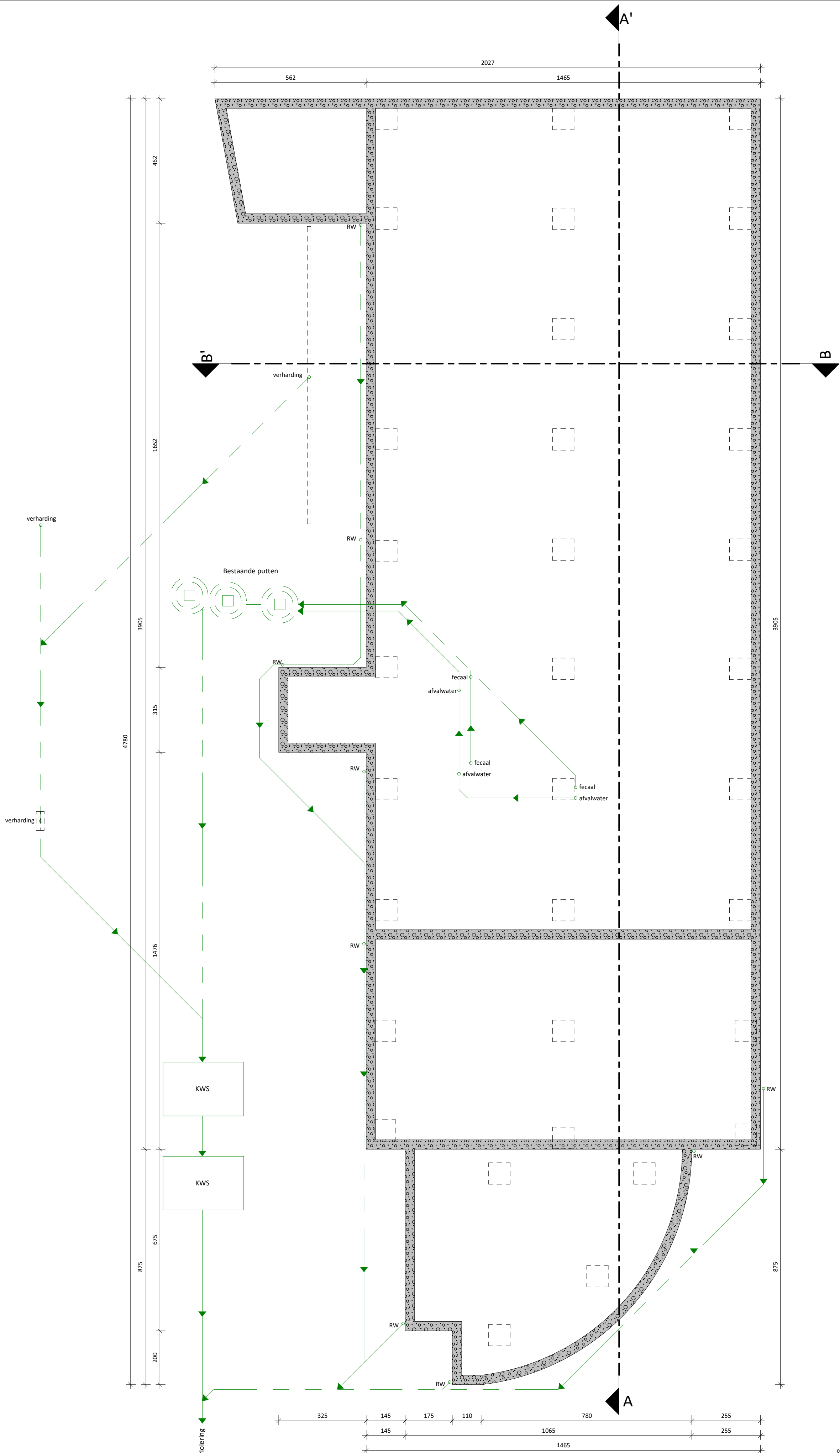
VT_Funderings- en rioleringsplan | Vergunde toestand | 1 : 100
