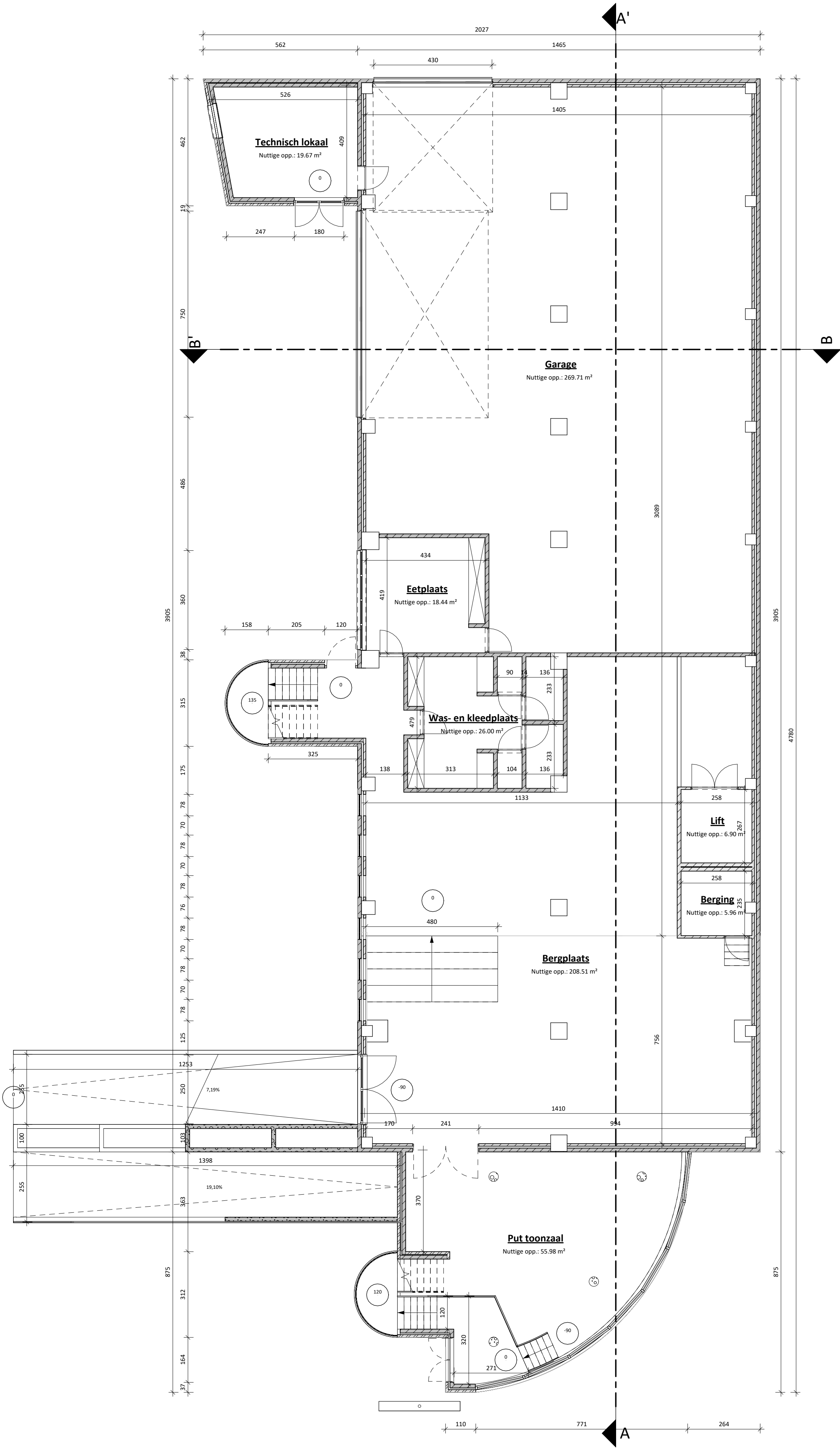
VT_Gelijkvloers | Vergunde toestand | 1 : 100
