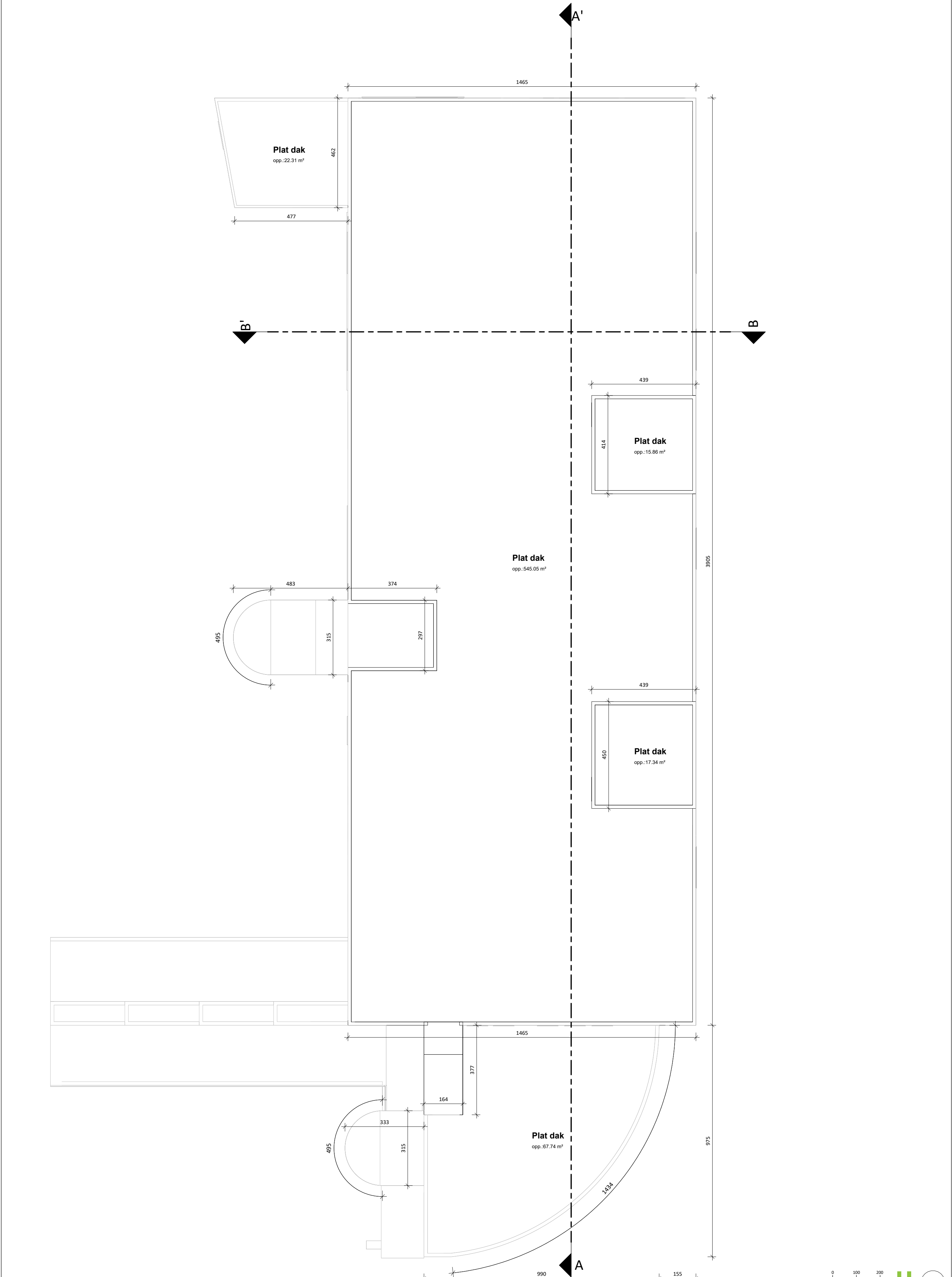
BT_Dakenplan | Bestaande toestand | 1 : 100
