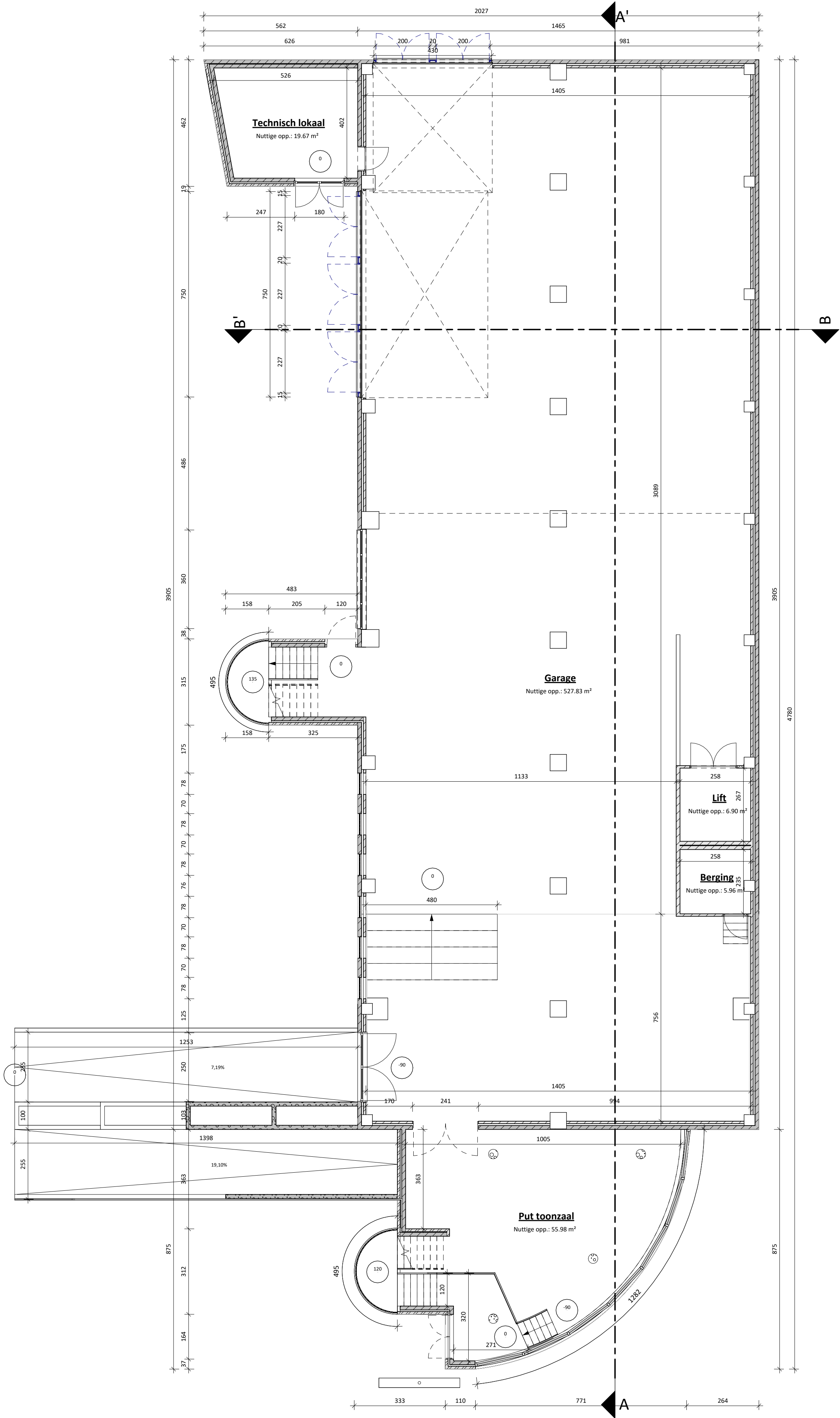
BT_Gelijkvloers | Bestaande toestand | 1 : 100
