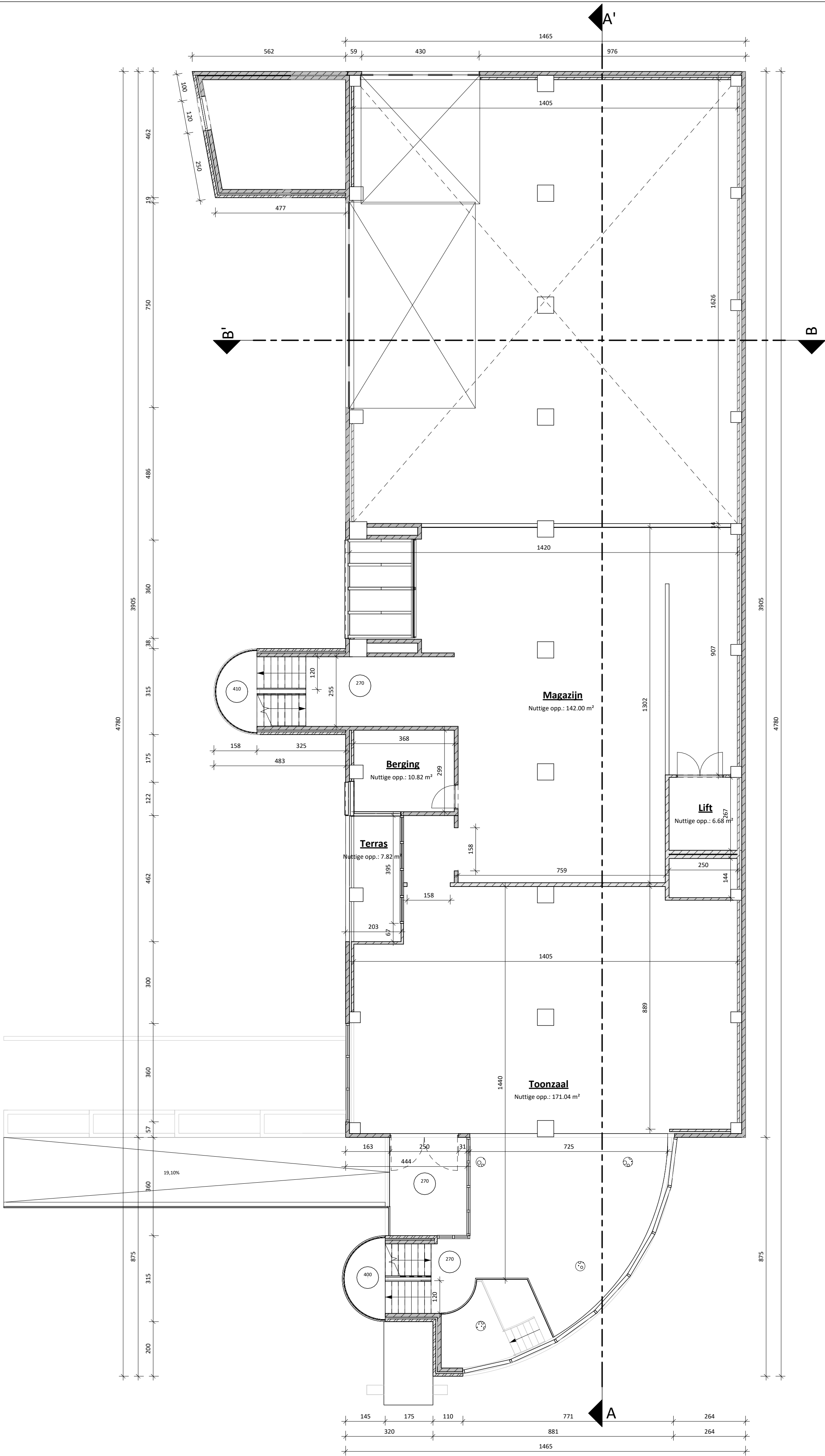
BT_Verdieping +1 | Bestaande toestand | 1 : 100
