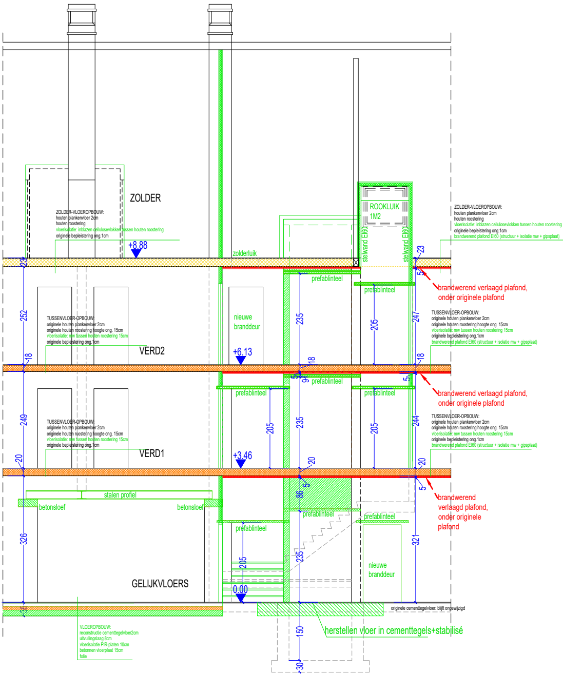
SNEDE GANG-LIFT
