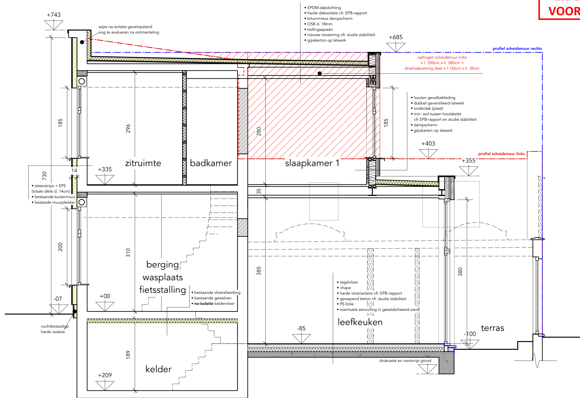
DOORSNEDE AB
