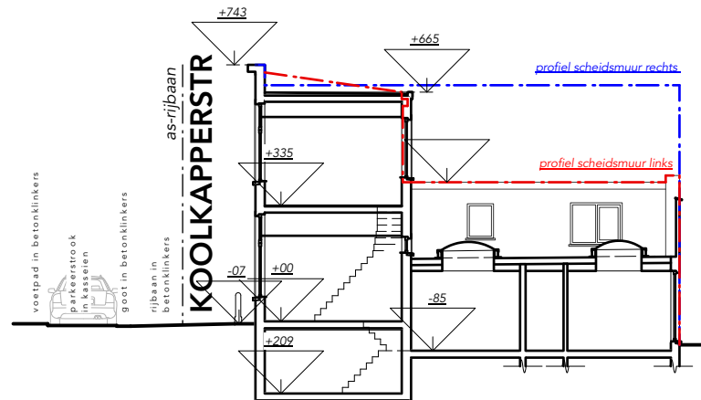
terreinprofiel
