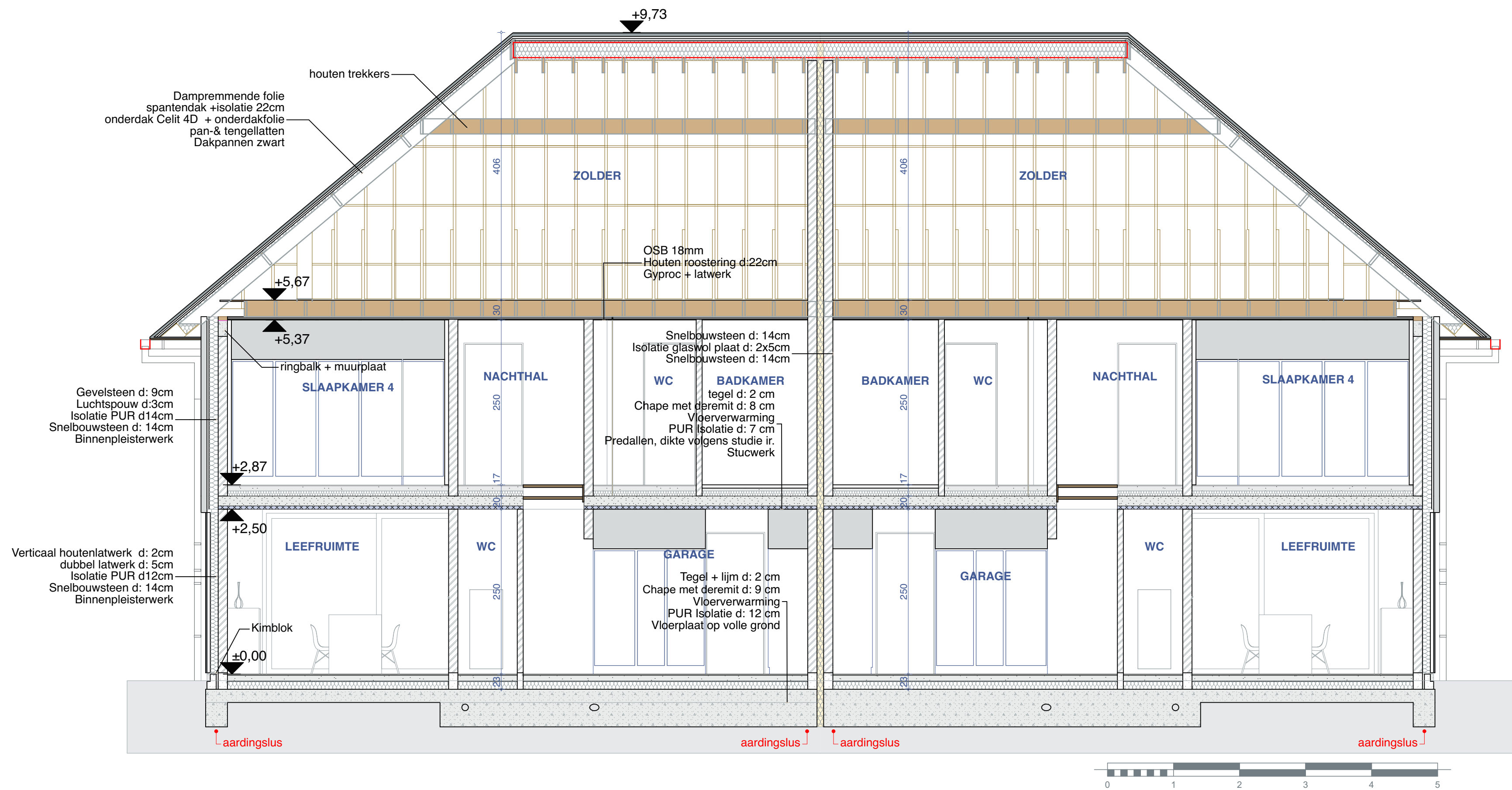
DOORSNEDE 02 Schaal 1/50
