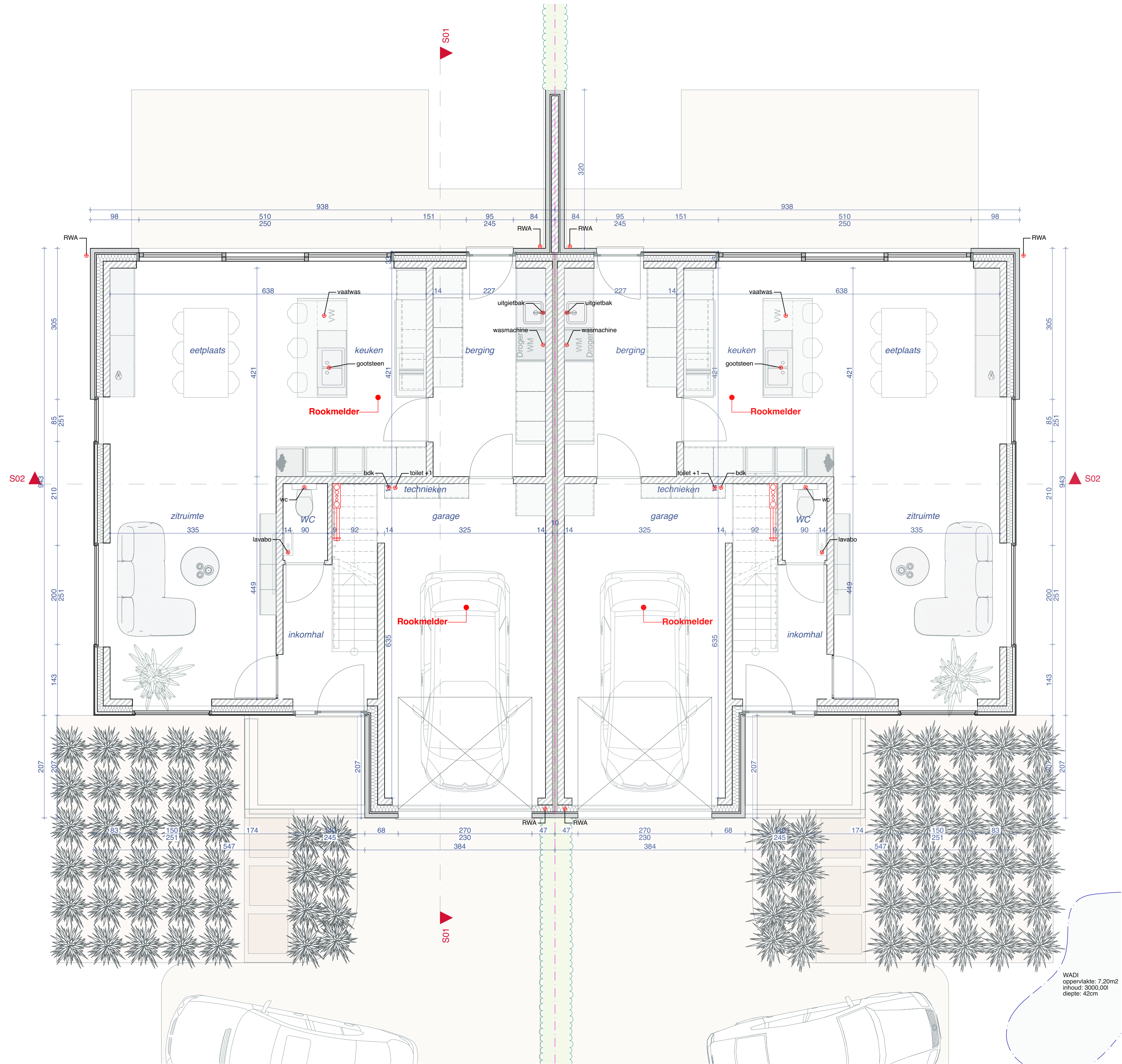
GRONDPLAN GELIJKVLOERS
