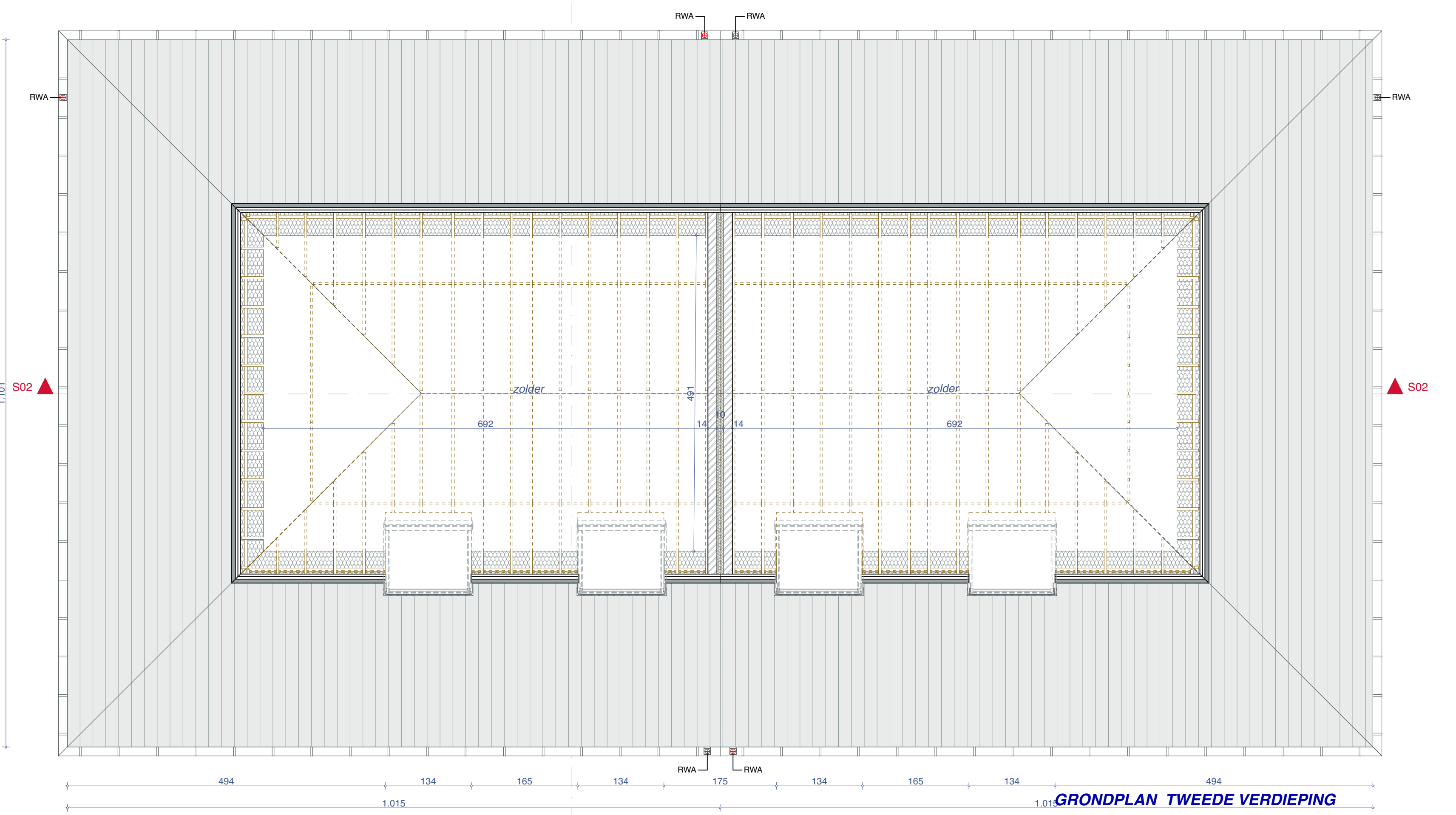
GRONDPLAN TWEEDE VERDIEPING
