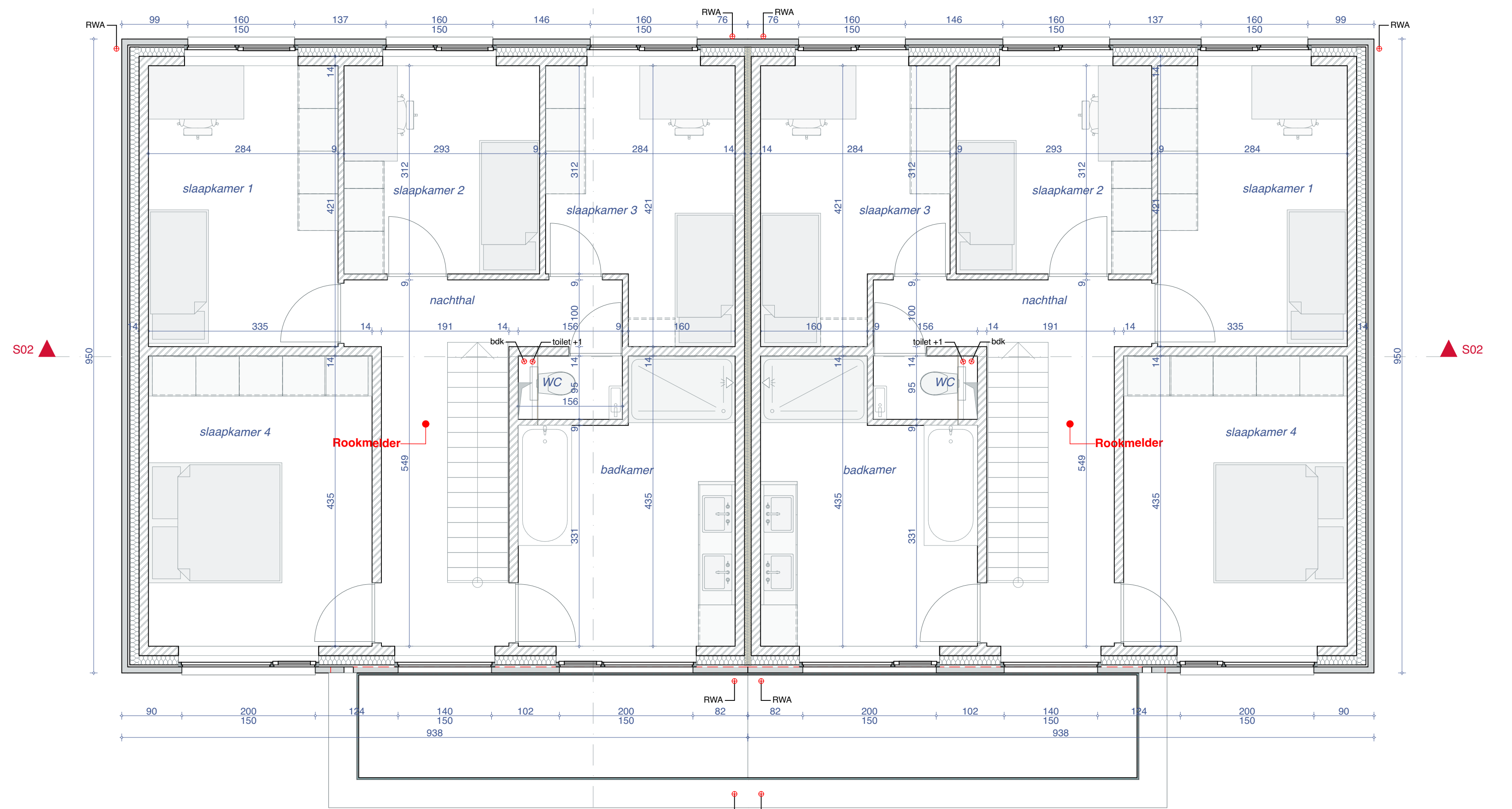
GRONDPLAN EERSTE VERDIEPING
