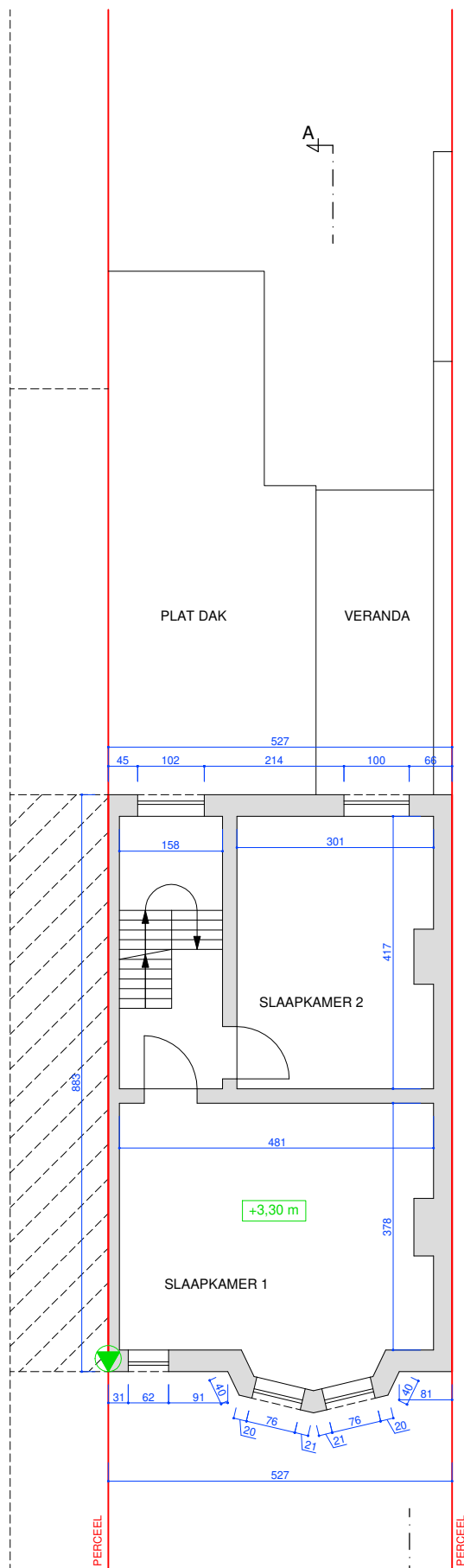
VERDIEPING 01 bestaande toestand
