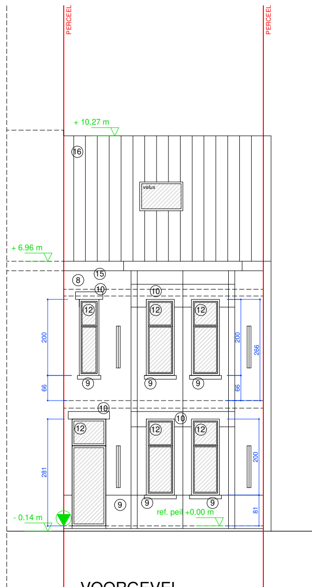
VOORGEVEL nieuwe toestand
