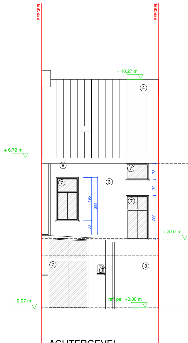
ACHTERGEVEL bestaande toestand
