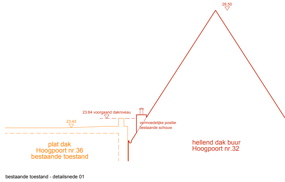
bestaande toestand - detailsnede 01
