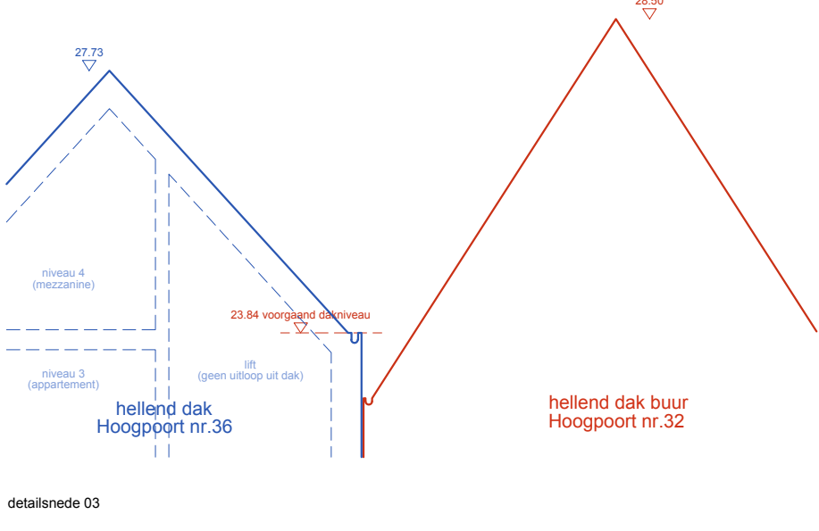
detailsnede 03
