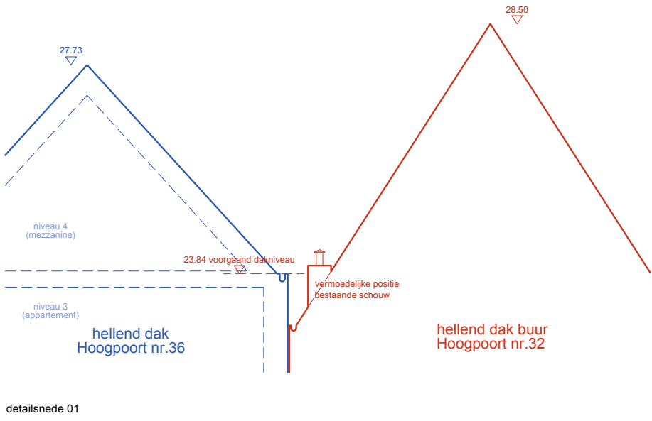
detailsnede 01
