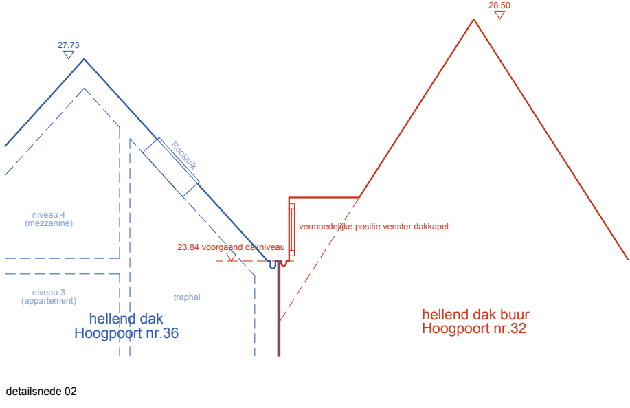
detailsnede 02
