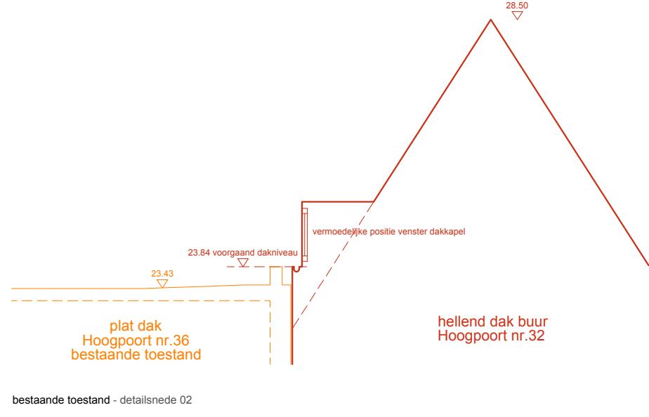
bestaande toestand - detailsnede 02
