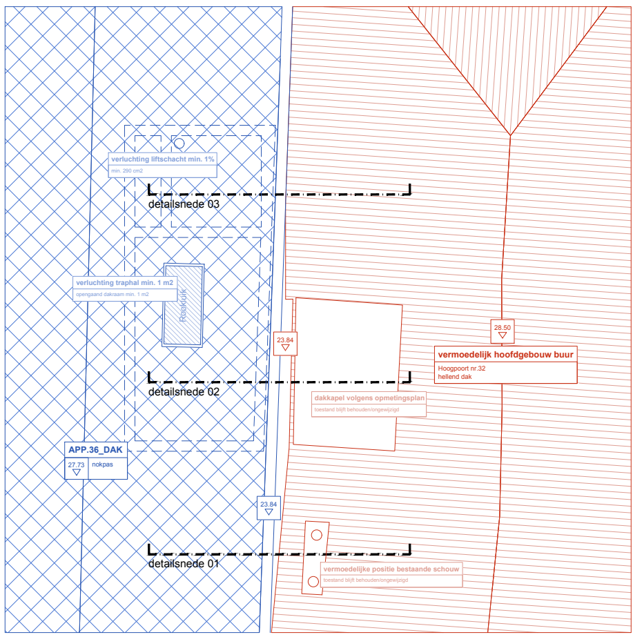
extractie dakplan thv dakkapel hoogpoort nr 32
