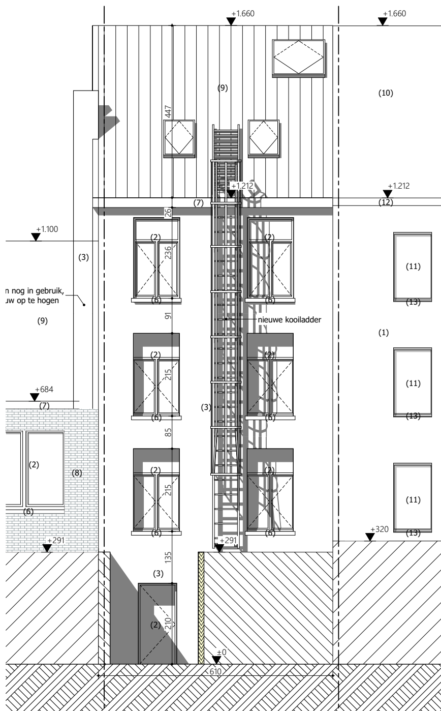
AG Achtergevel - nieuwe toestand 1:100
