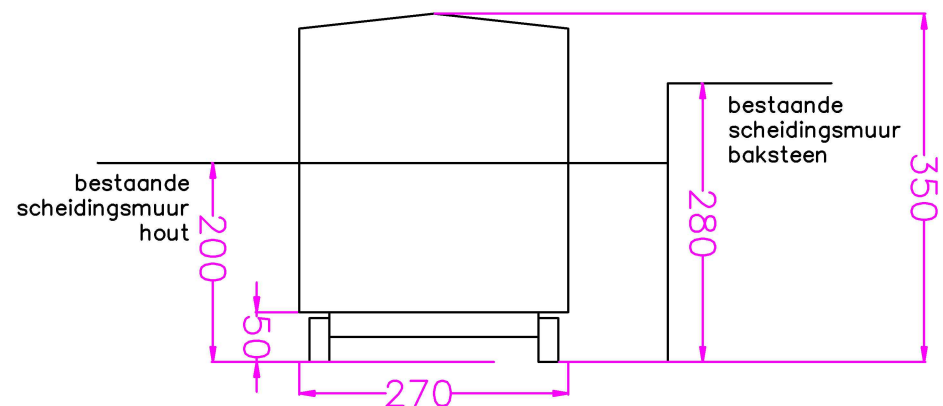
Zijaanzicht rechts
