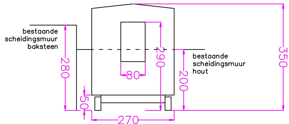
Zijaanzicht links
