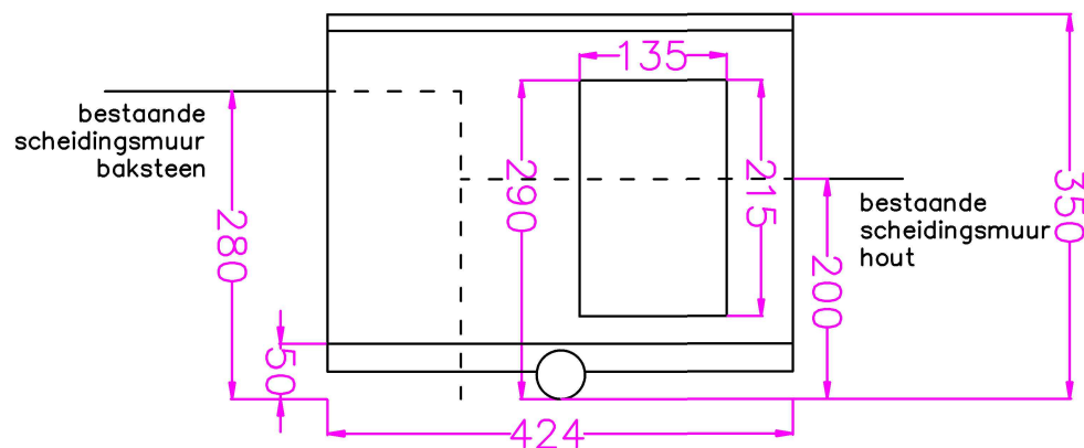
Vooraanzicht
