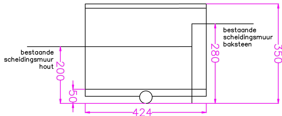
Achteraanzicht
