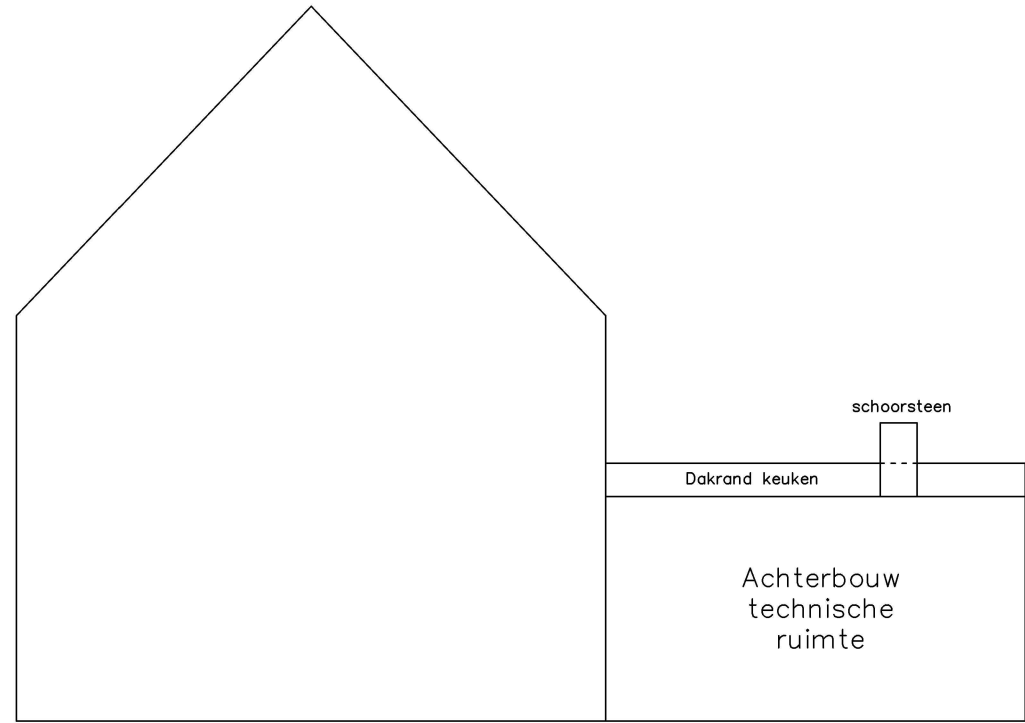
Zijaanzicht rechts
