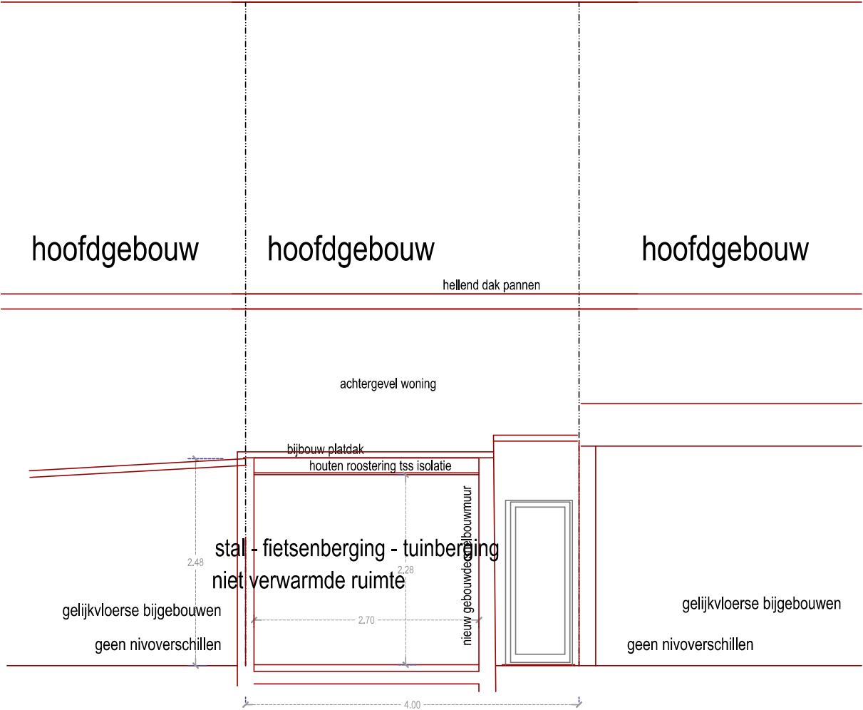
doorsnede AA
