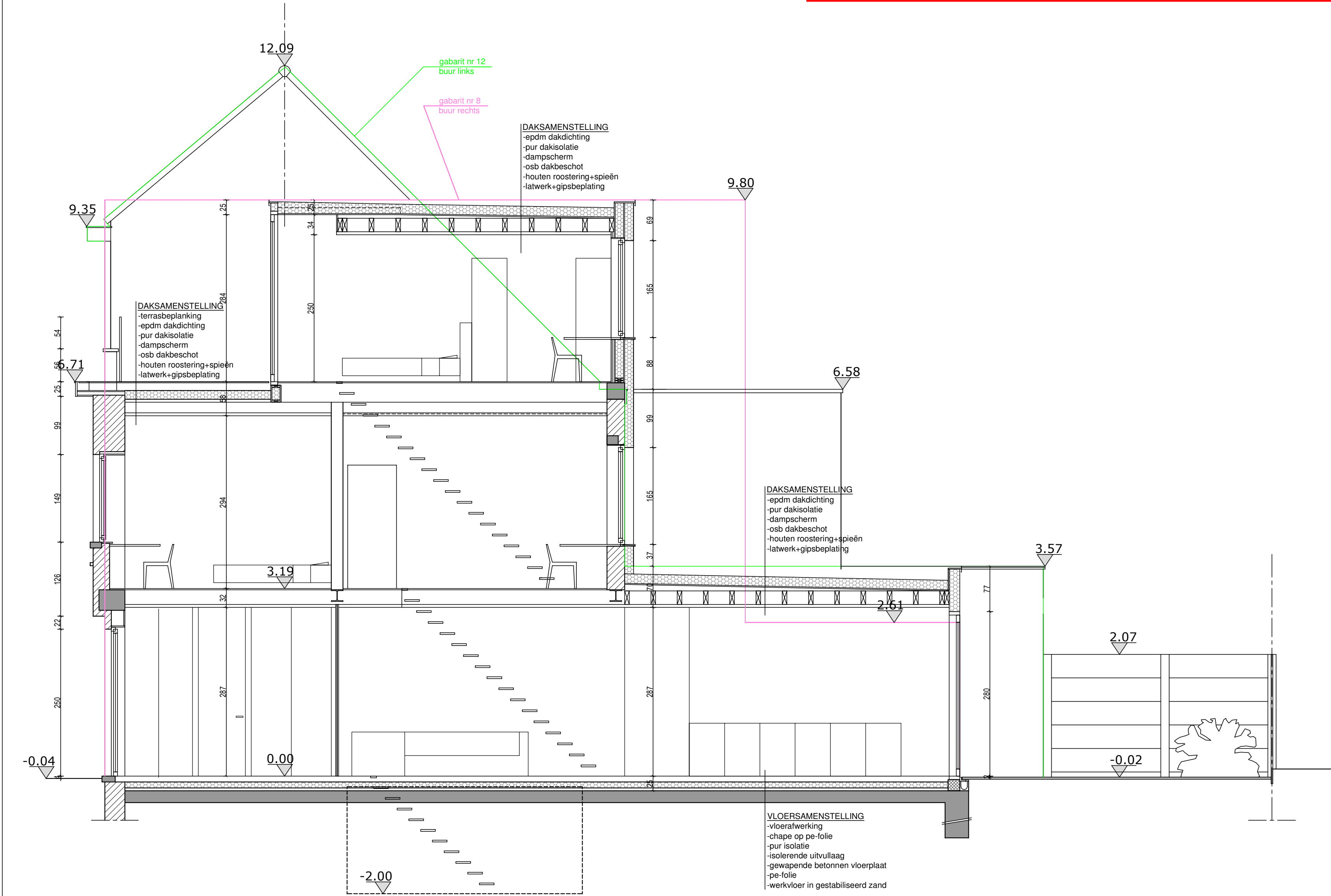
DOORSNEDE A NIEUWE TOESTAND
