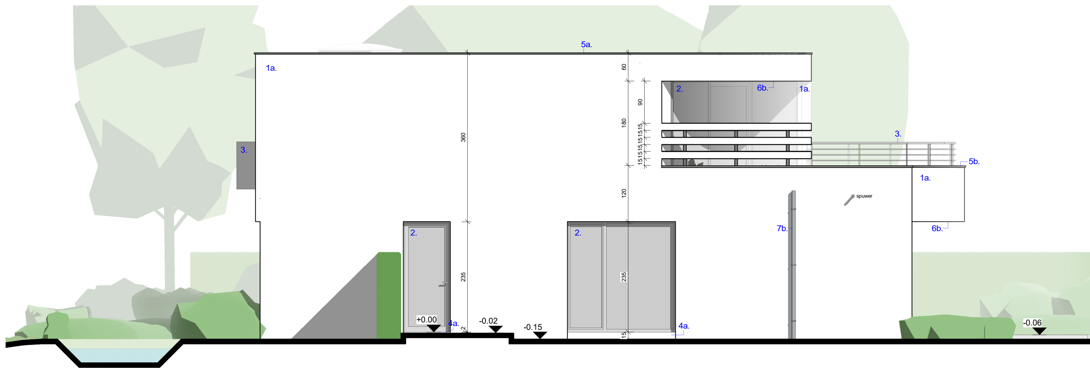
1 .Zijgevel rechts 1 : 50
