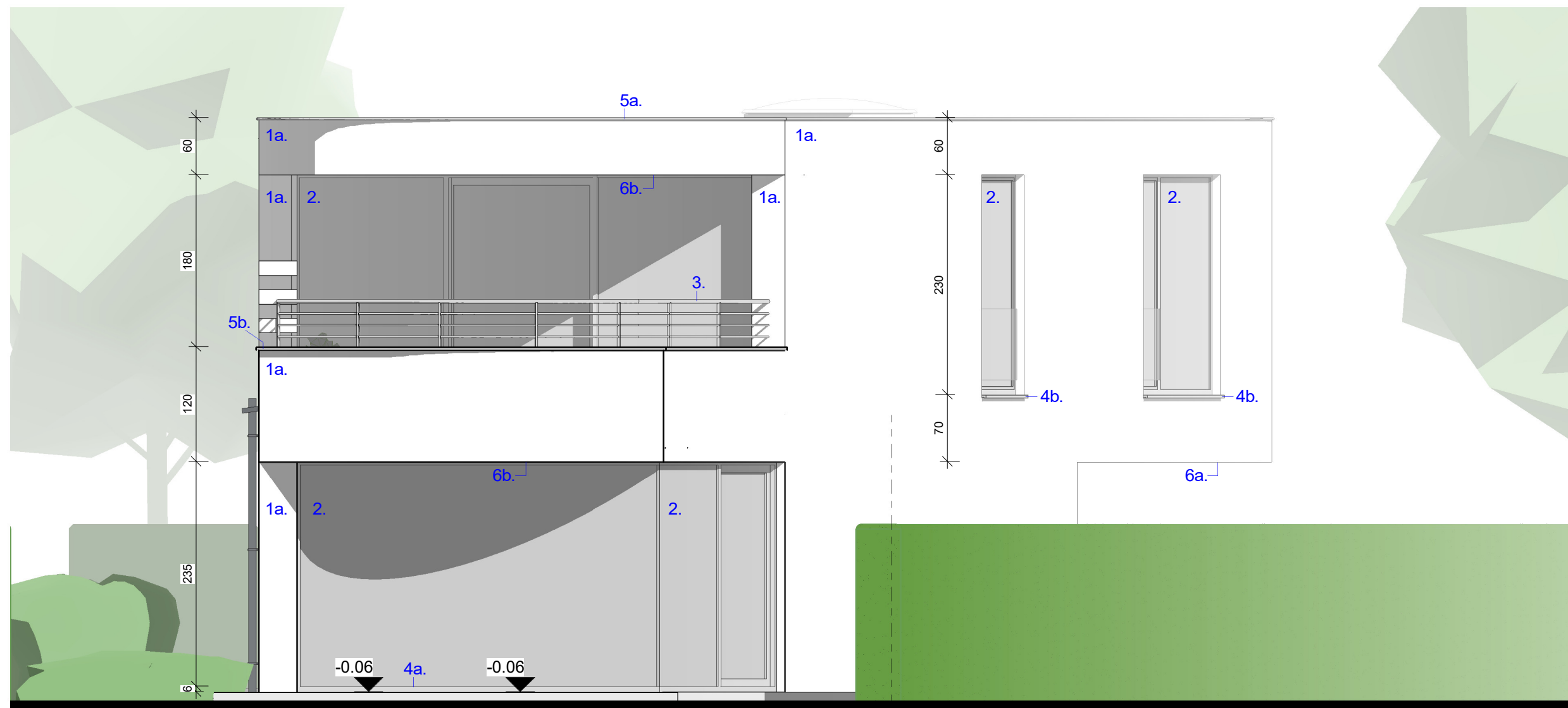
1 .Achtergevel 1 : 50
