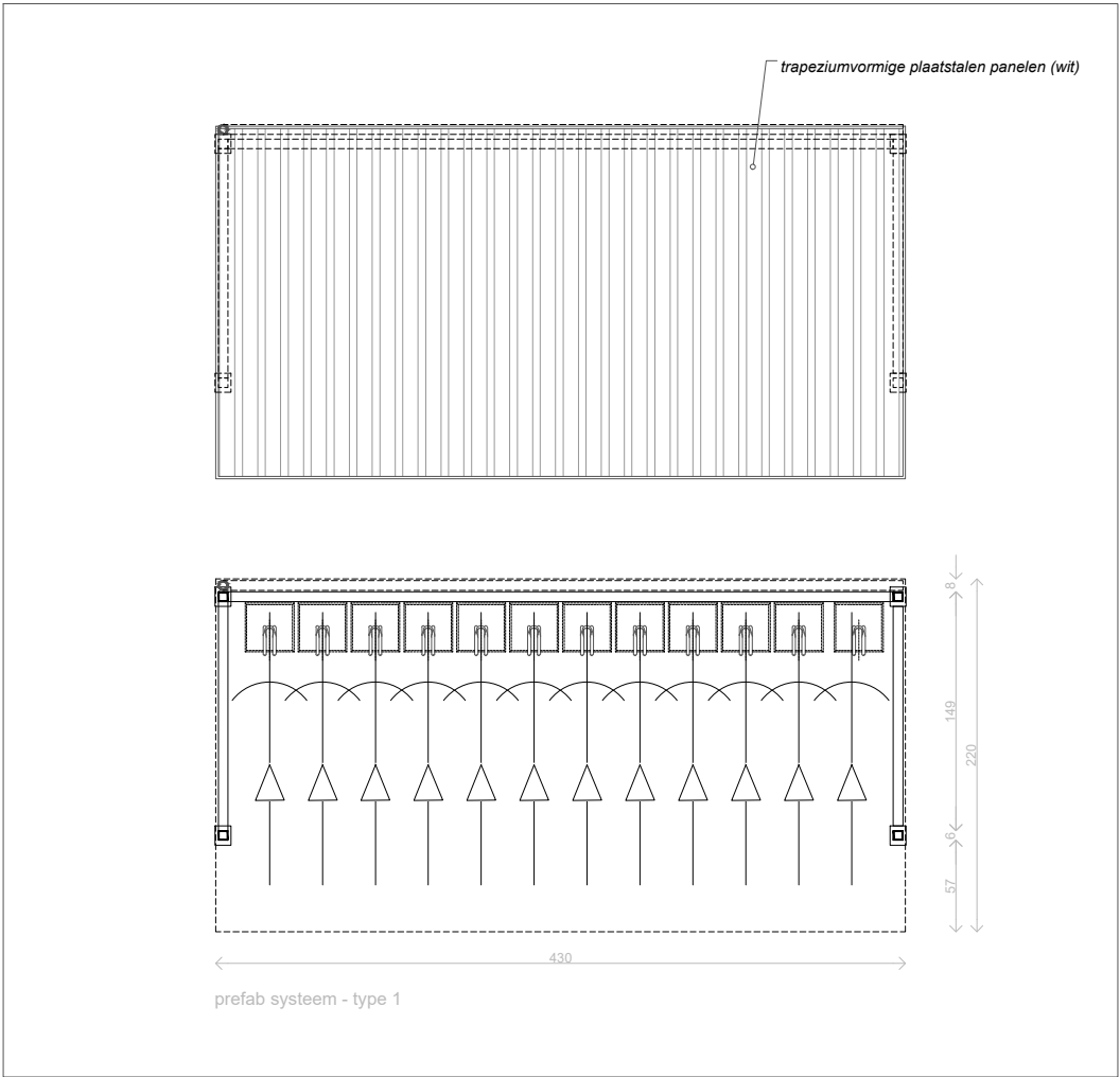
plan - bovenaanzicht 1/50
