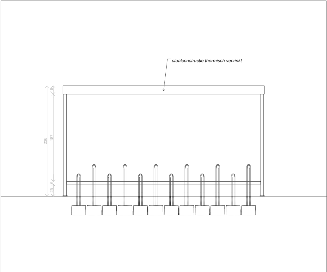
vooraanzicht 1/50
