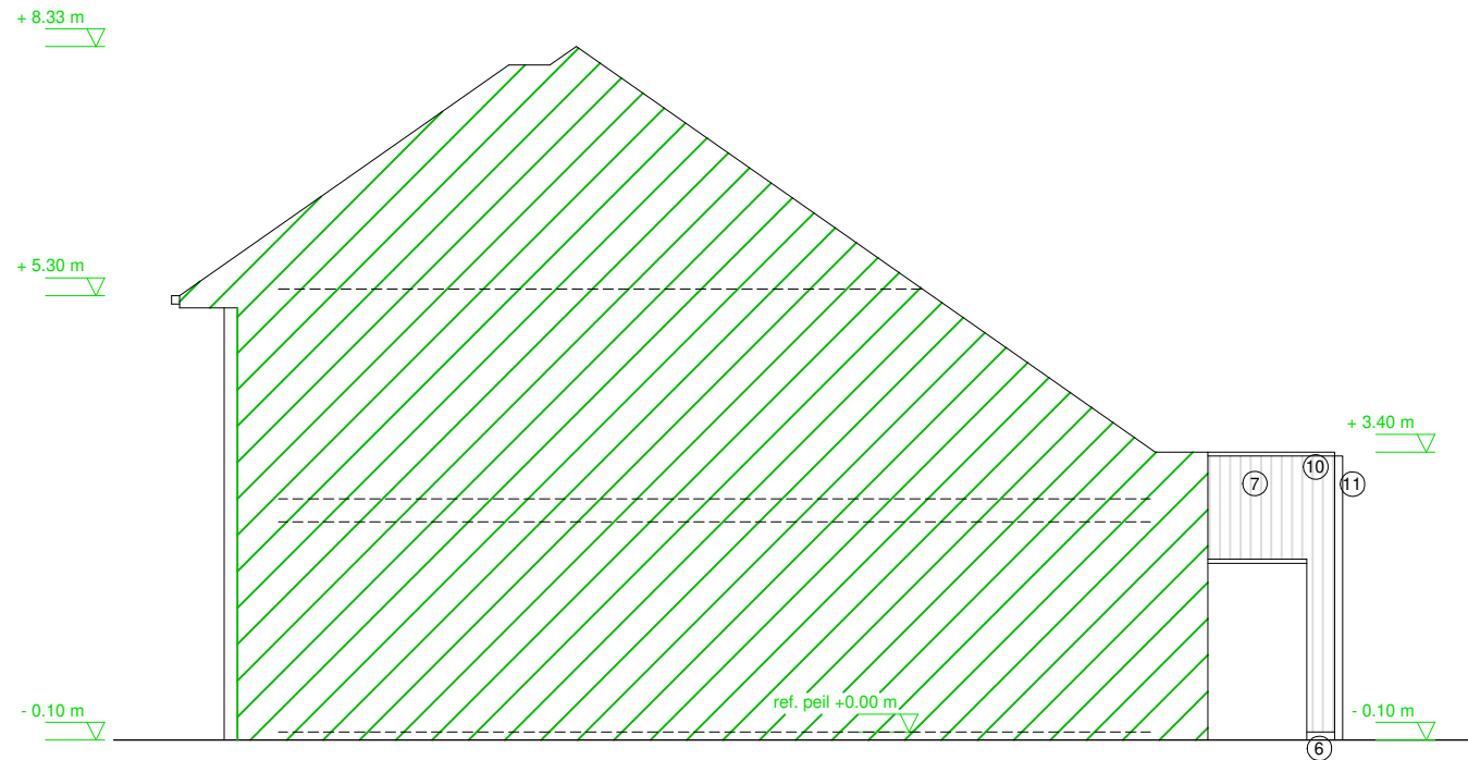
ZIJGEVEL RECHTS nieuwe toestand
