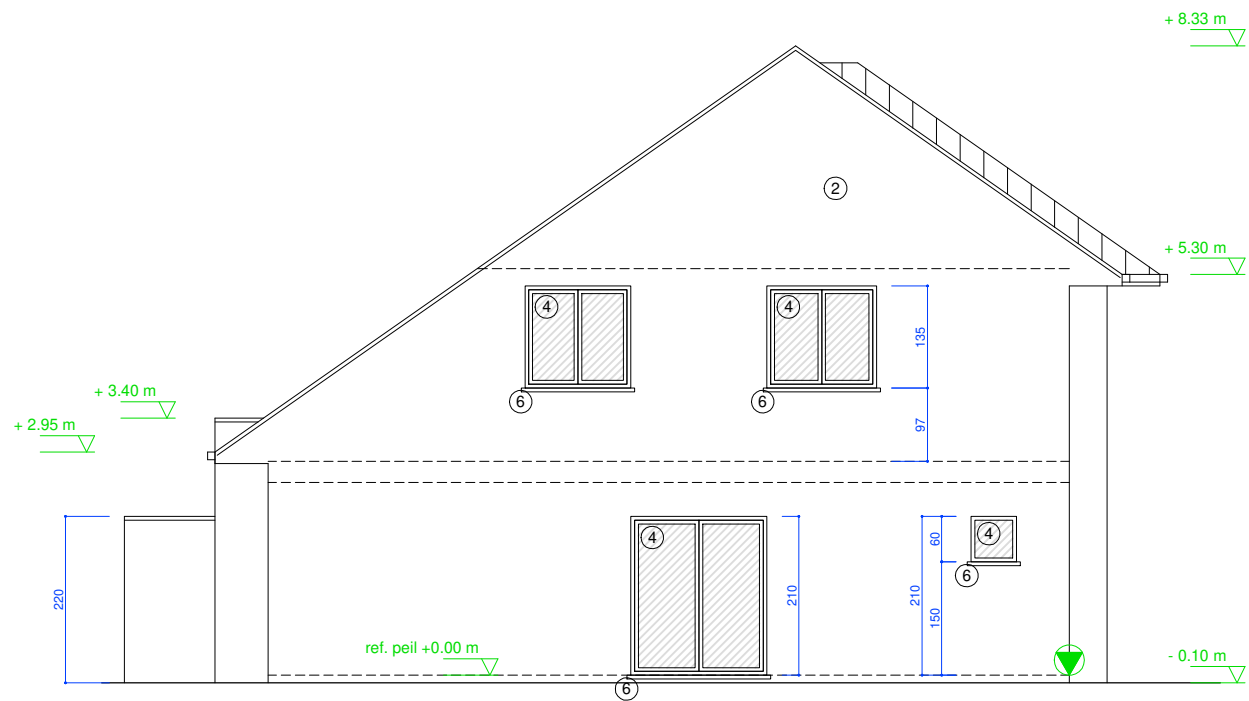
ZIJGEVEL LINKS bestaande toestand
