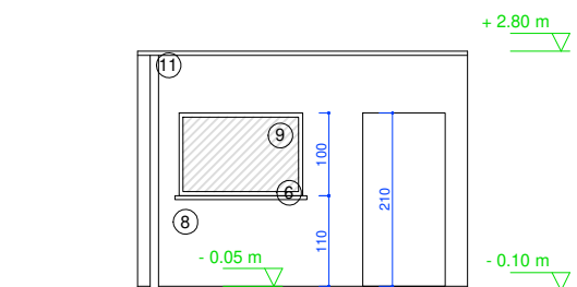
VOORGEVEL tuinhuis
