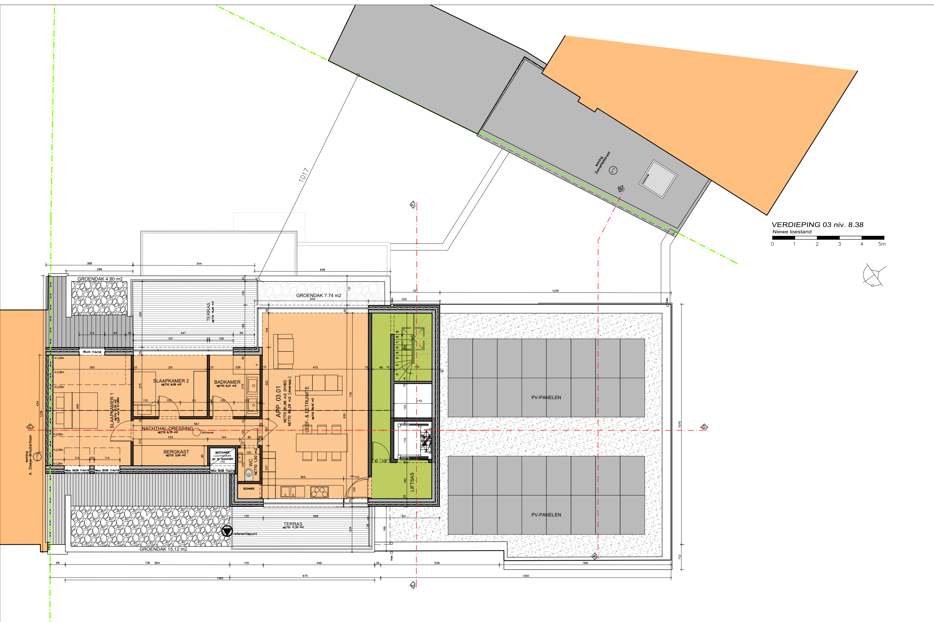
PLAN VERDIEPING 3 TOESTAND NA VERBOUWING
