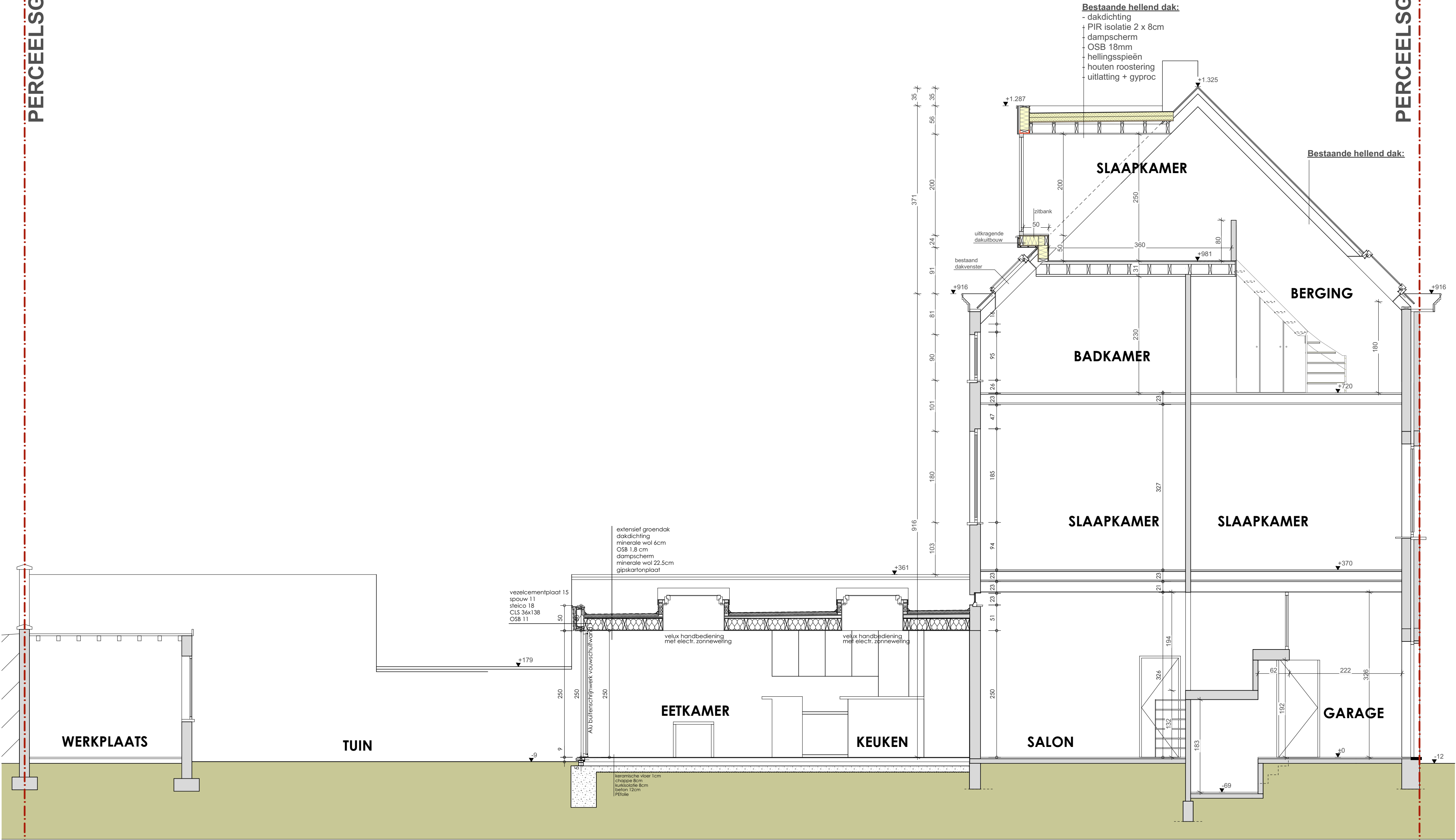
DOORSNEDE A NIEUWE TOESTAND - schaal 1/50
