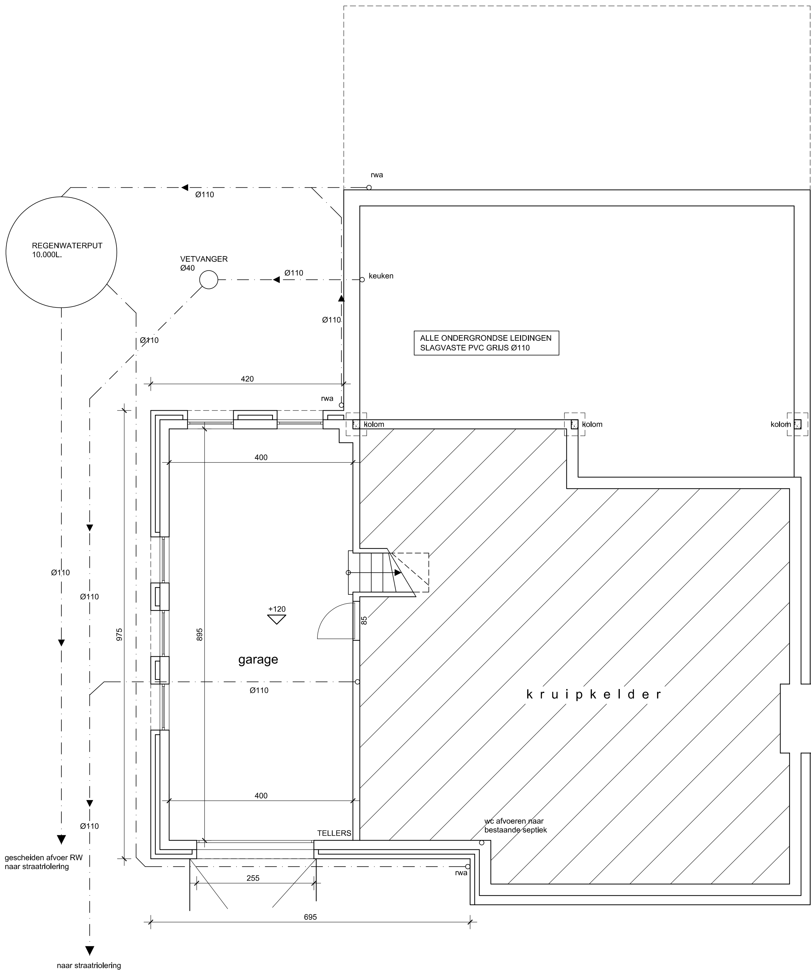
GARAGE - KRUIPKELDER FUNDERING - RIOLERING 1/50
