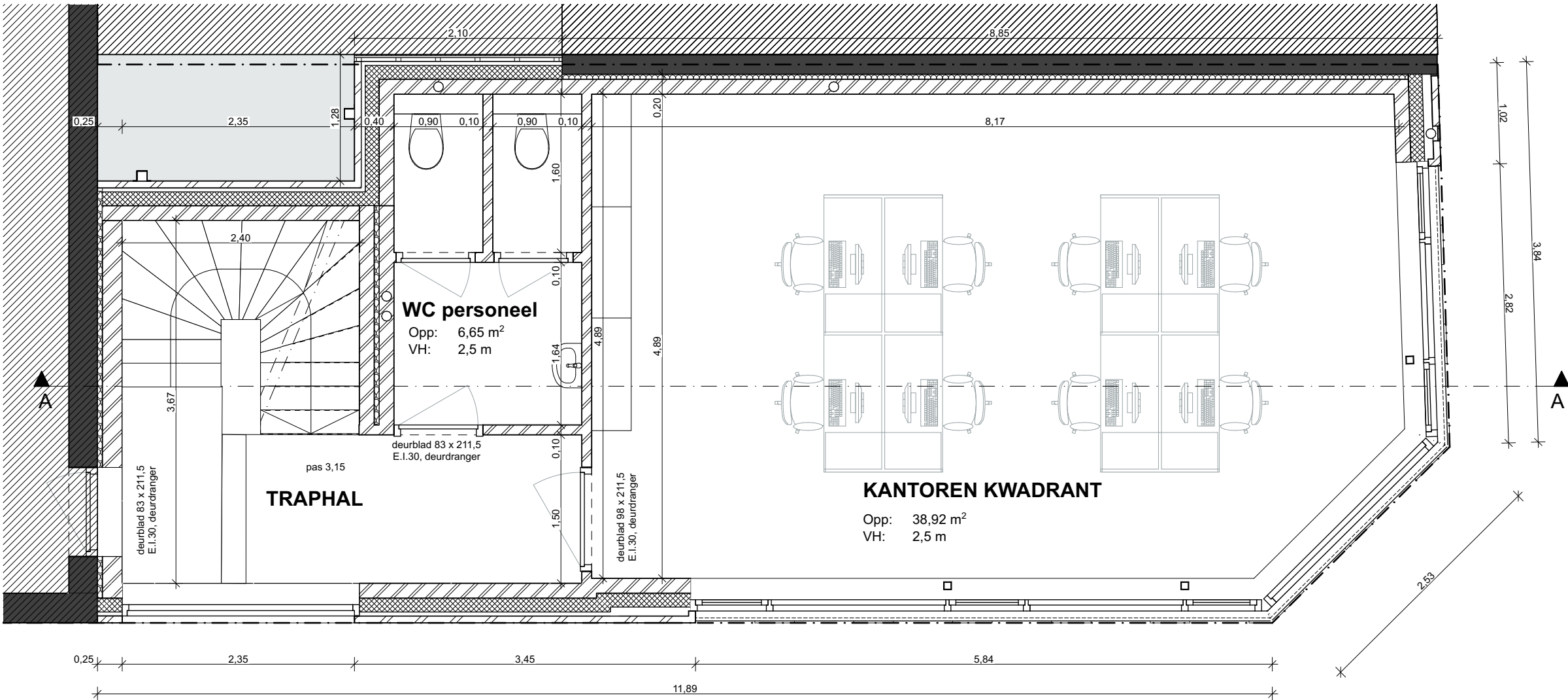
PLAN VERDIEPING 1 schaal 1/50, maataanduiding in meter.
