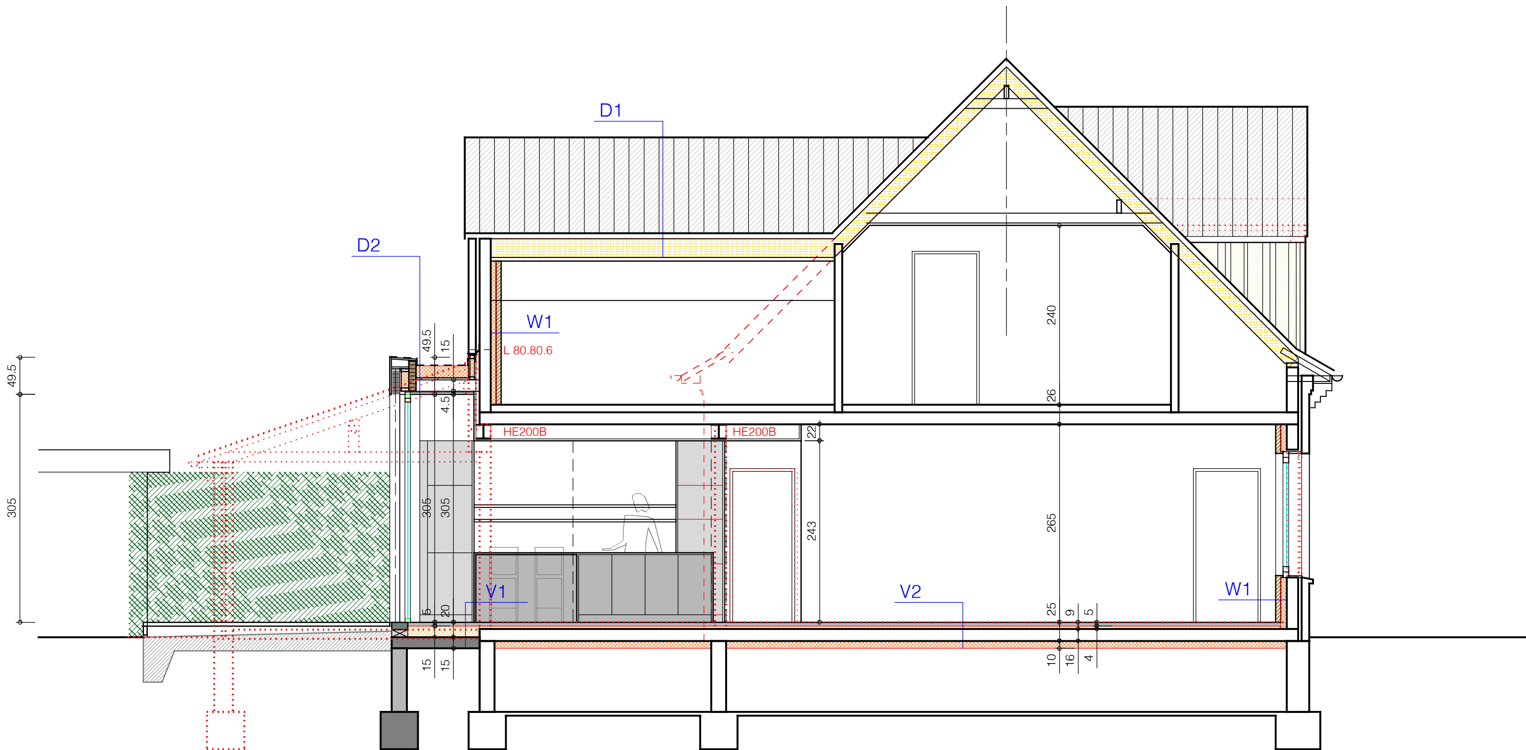
snede 1
